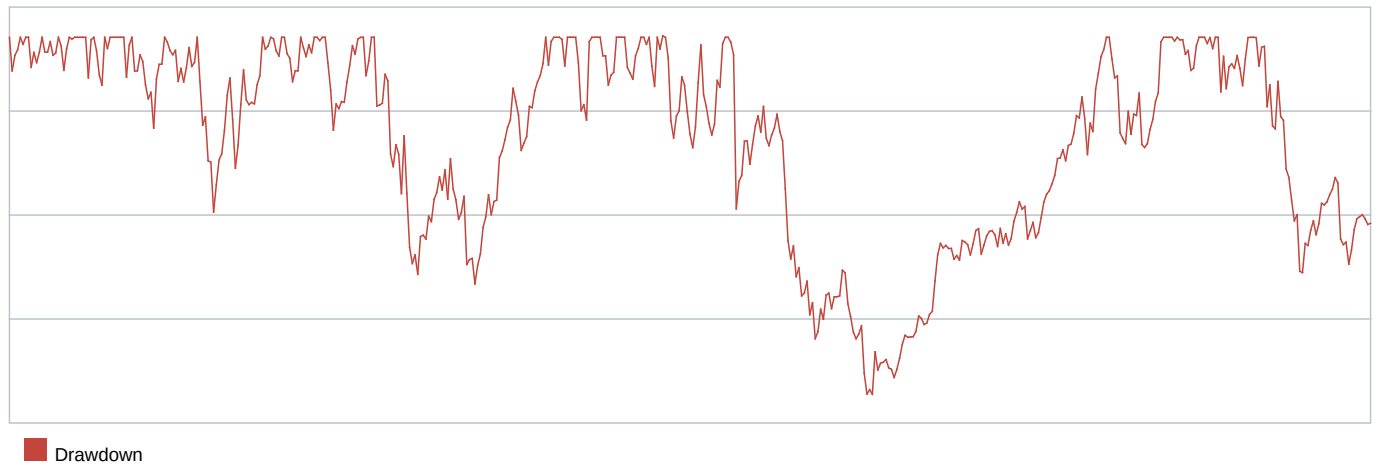
ARMS Drawdown
