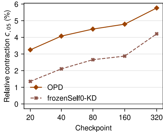
(d) Matched support, different target
