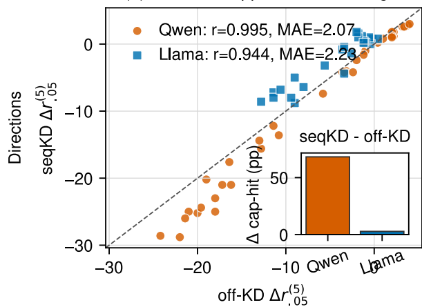
(d) Matched support, different target
