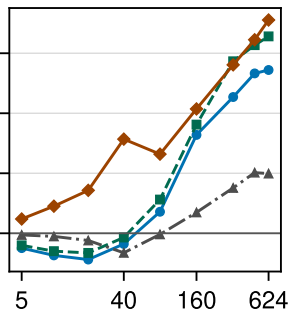
Llama / MMLU-Pro
