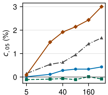
Llama / General
