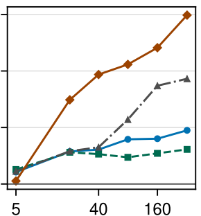
Llama / IFEval
