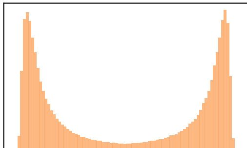
softsign
