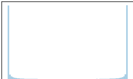
tanh
