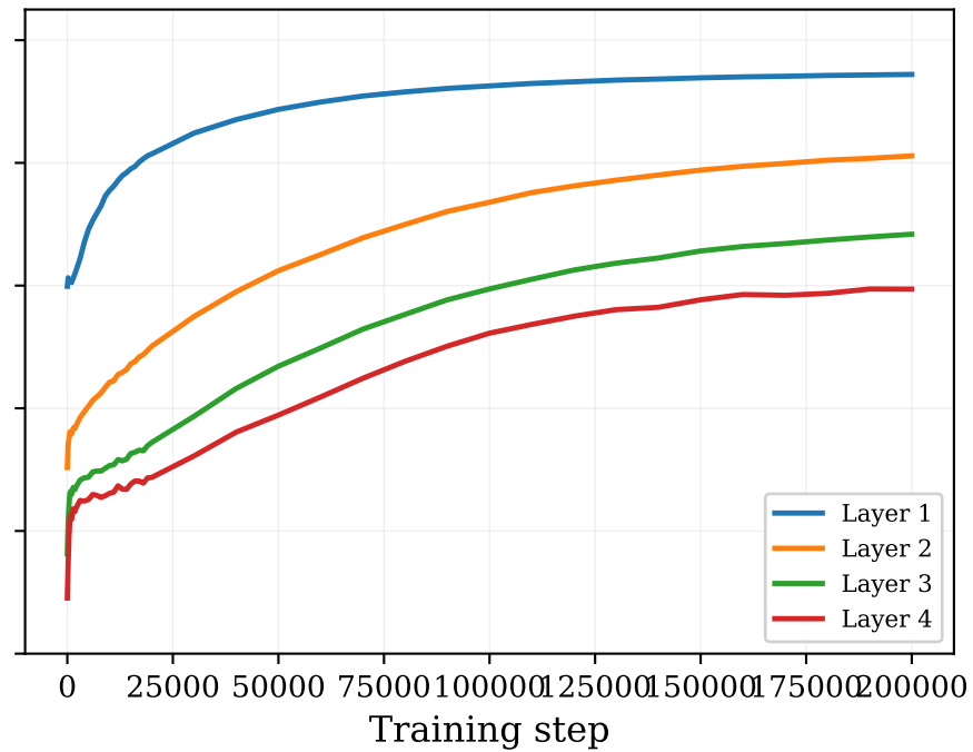
softsign
