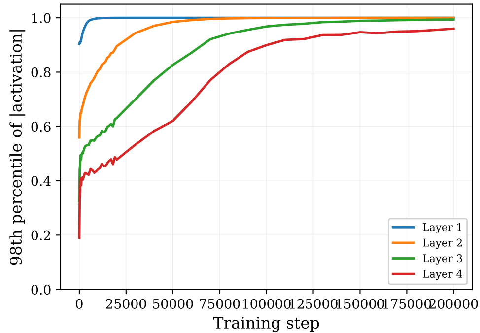
tanh
