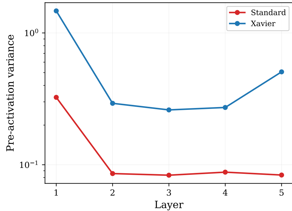
sigmoid
