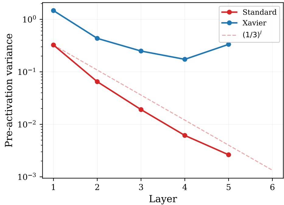
tanh
