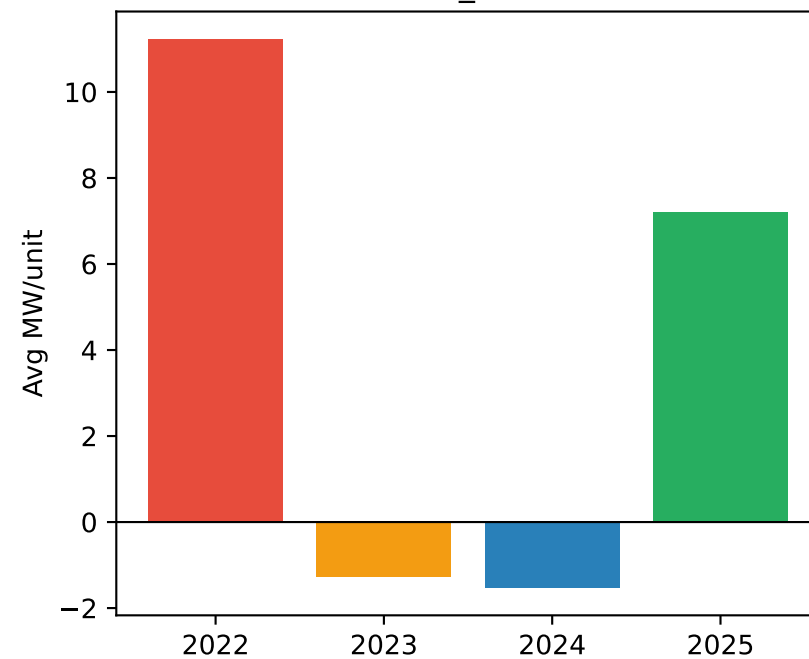
cloud_cover
