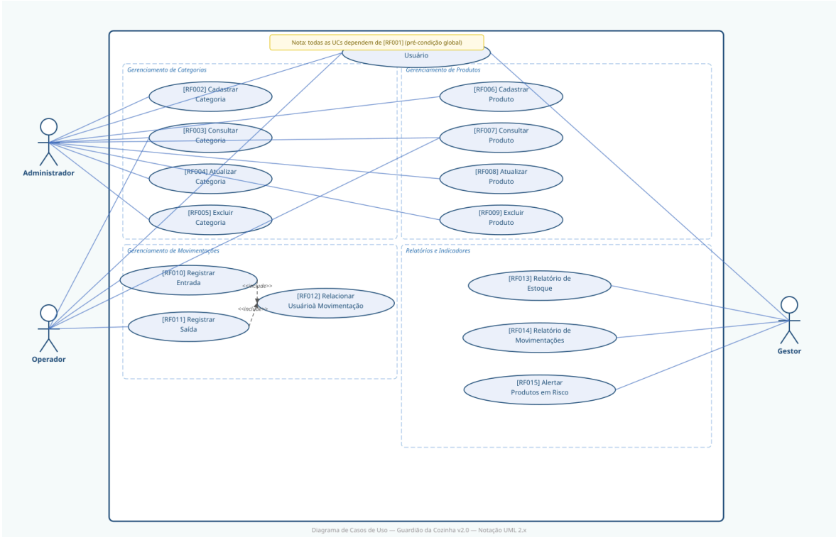
Figura 1 — Diagrama de Casos de Uso do Guardião da Cozinha (Notação UML 2.x)
