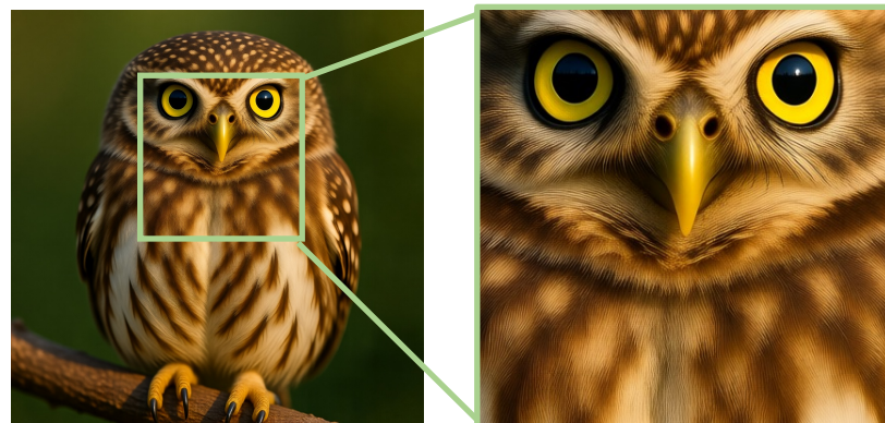
DMD2
