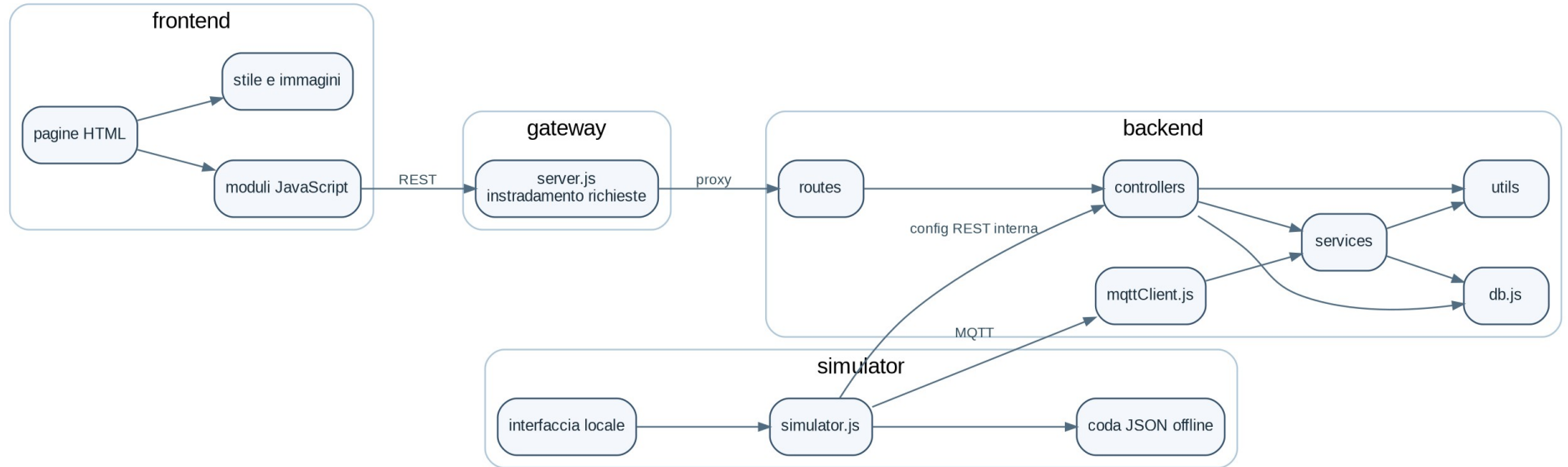
Figura 4 – Diagramma dei package
