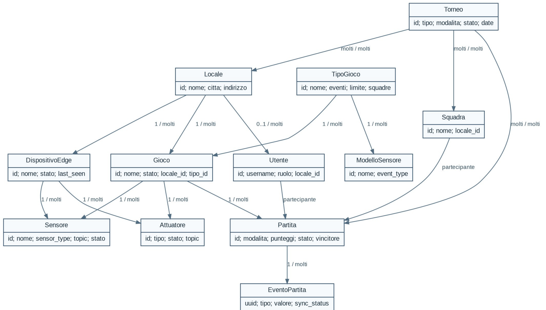
Figura 3 – Diagramma delle classi del dominio
