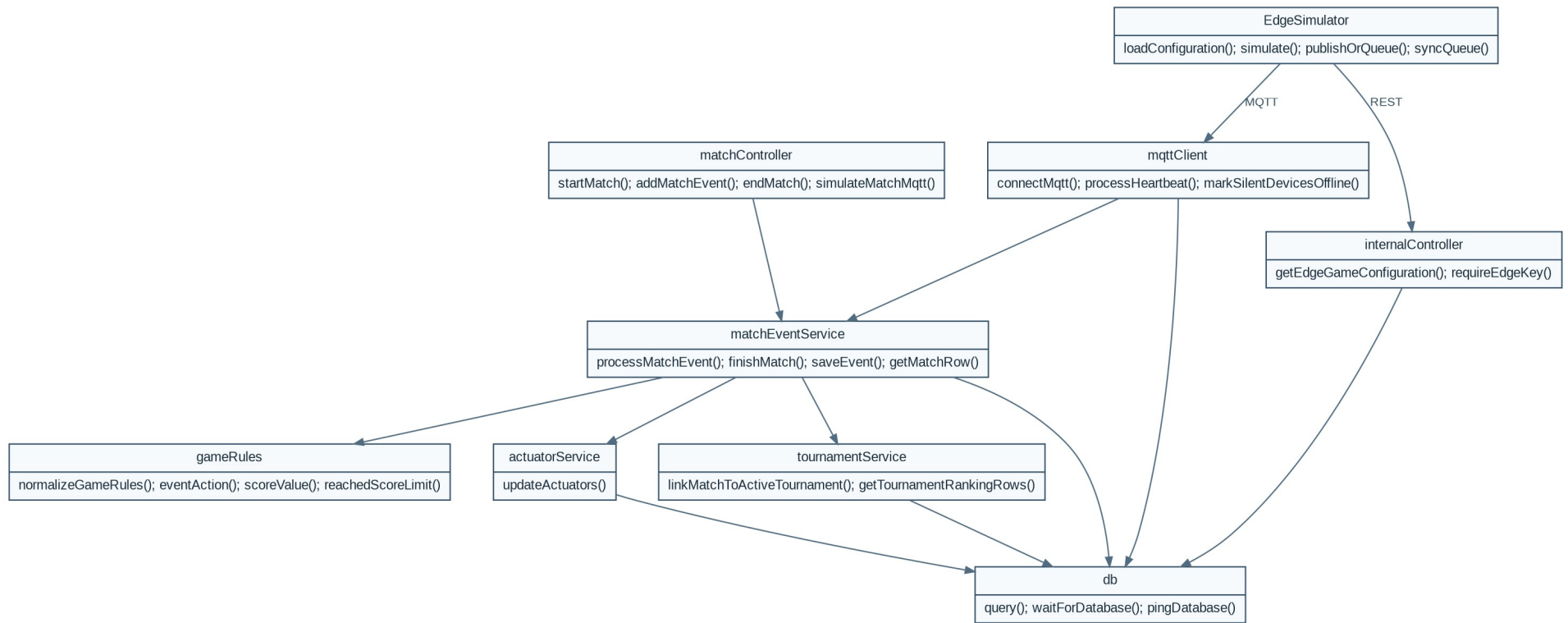
Figura 5 – Classi e moduli di implementazione
