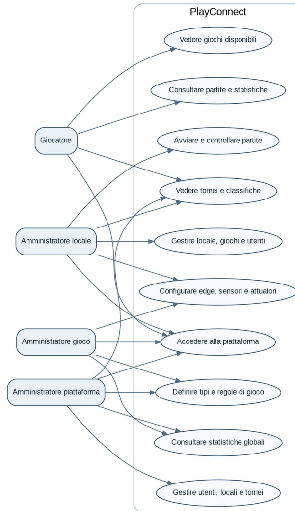
Figura 1 – Diagramma dei casi d'uso
