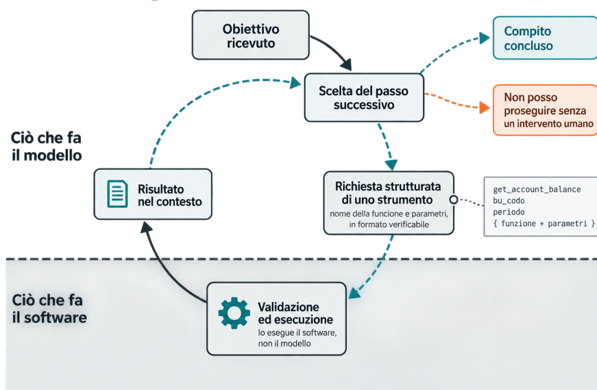
Figura 4: Il ciclo agentic
