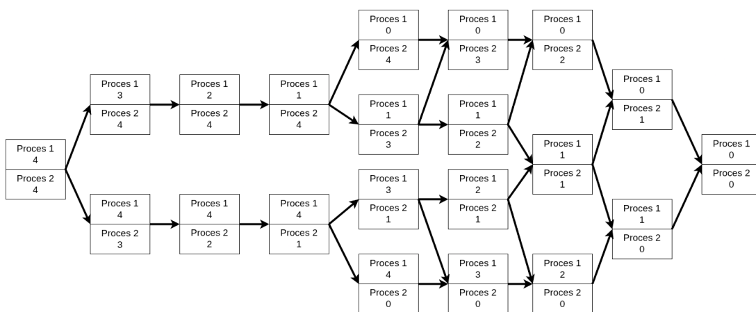
Obr. 3: Ochrana kritickej sekcie pomocou mutexu
