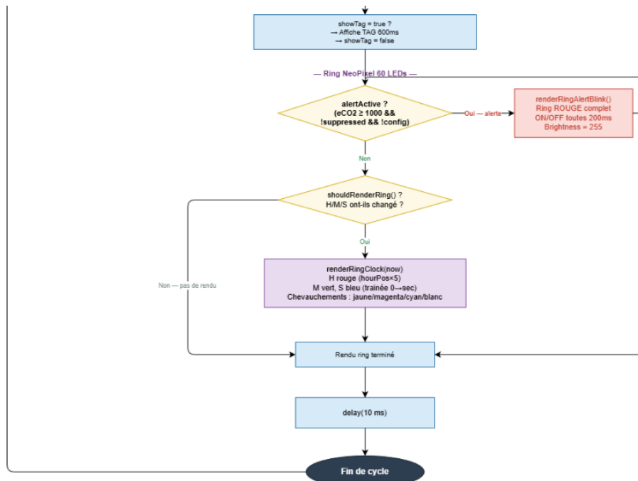
Figure 27 Image du diagramme de flux du code partie 3
