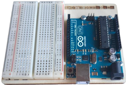
Figure 2 Photo de l'Arduino et de sa Breadboard prise à la main
