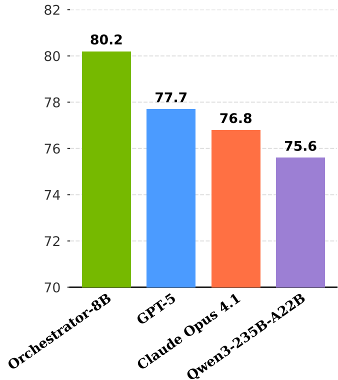
Tau2-Bench
