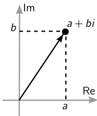
Figura 1. Il piano complesso.
