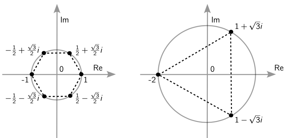
Figura 5. Le radici seste di 1, cioè le soluzioni di z^6 = 1 , sono i vertici di un esagono regolare centrato nell'origine con un vertice in 1 (sinistra). Le soluzioni di z^3 = -8 sono i vertici di un triangolo equilatero centrato nell'origine e di raggio \sqrt[3]{8} = 2 (destra).
