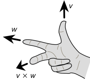
Figura 9. La regola della mano destra.
