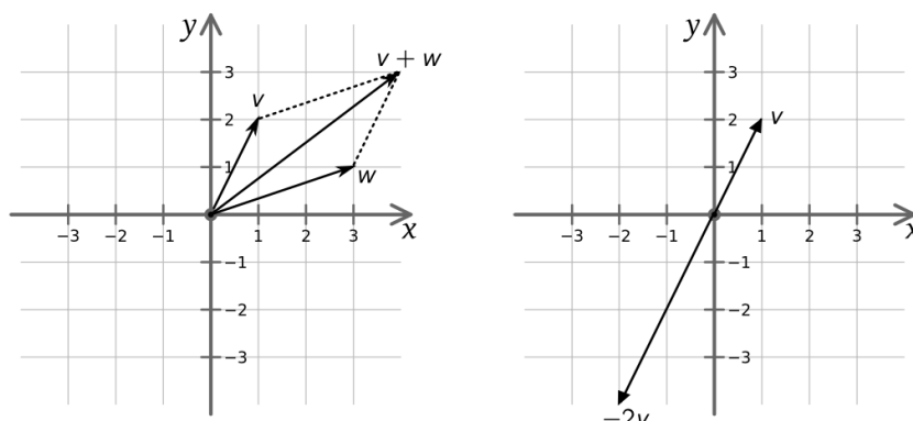
Figura 6. La somma v + w di due vettori v, w \in \mathbb{R}^2 e la moltiplicazione di un vettore v per uno scalare \lambda (qui \lambda = -2 ).
