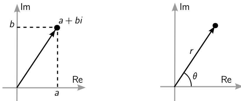
Figura 3. Il piano complesso (sinistra) e le coordinate polari (destra).
