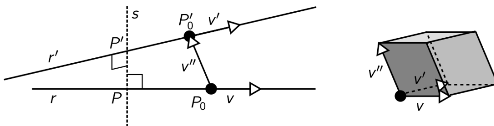
Figura 11. La distanza fra due rette sghembe è la lunghezza del segmento PP' ortogonale ad entrambe.
