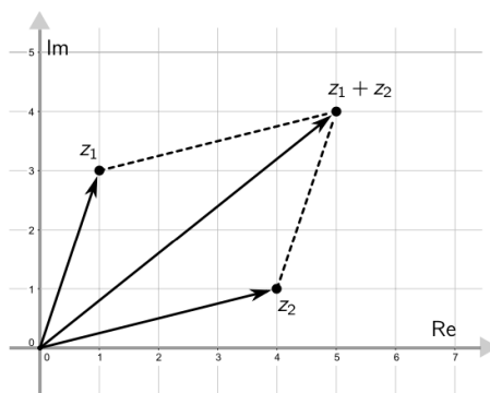
Figura 2. La somma z_1 + z_2 di due numeri complessi z_1 e z_2 può essere calcolata con la regola del parallelogramma. Qui z_1 = 1 + 3i , z_2 = 4 + i e quindi z_1 + z_2 = 5 + 4i .
