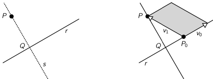
Figura 10. La distanza fra P e la retta r è la lunghezza del segmento PQ ortogonale a r .
