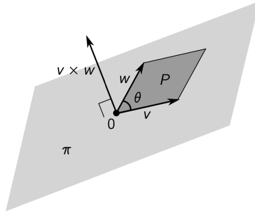
Figura 8. Il modulo \|v \times w\| è pari all'area del parallelogramma P con lati v e w contenuto nel piano \pi = \text{Span}(v, w) .
