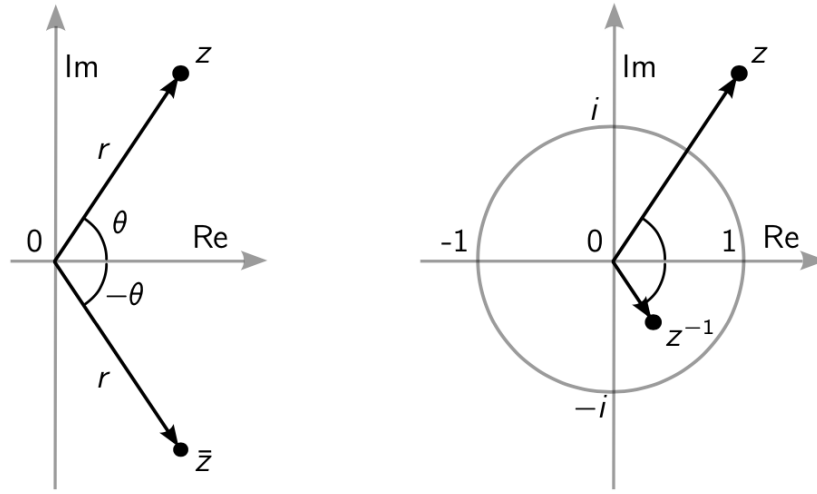
Figura 4. Il coniugio \bar{z} di z si ottiene specchiando z lungo l'asse reale (sinistra). L'inverso z^{-1} di z ha argomento -\vartheta opposto a quello \vartheta di z e modulo |z^{-1}| inverso rispetto a |z| . La circonferenza unitaria è mostrata in figura (destra).
