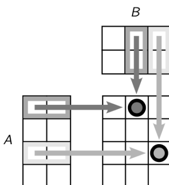
Figura 7. Il prodotto riga per colonna AB .
