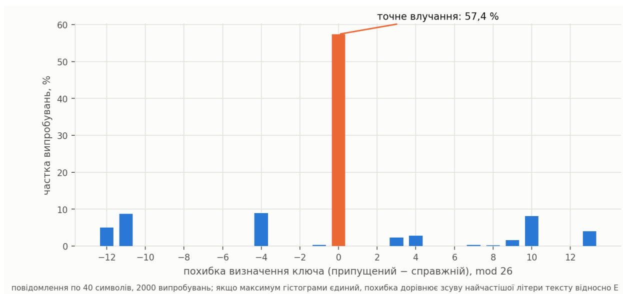
Рисунок 3.8 – Розподіл похибки найвнього правила визначення ключа
