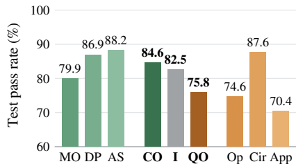
(d) Mini-SWE-Agent · All
