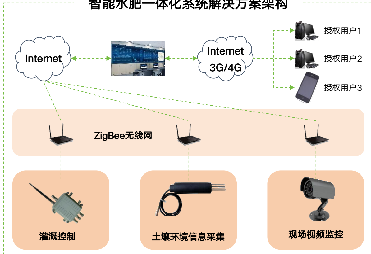
智能水肥一体化系统解决方案架构
