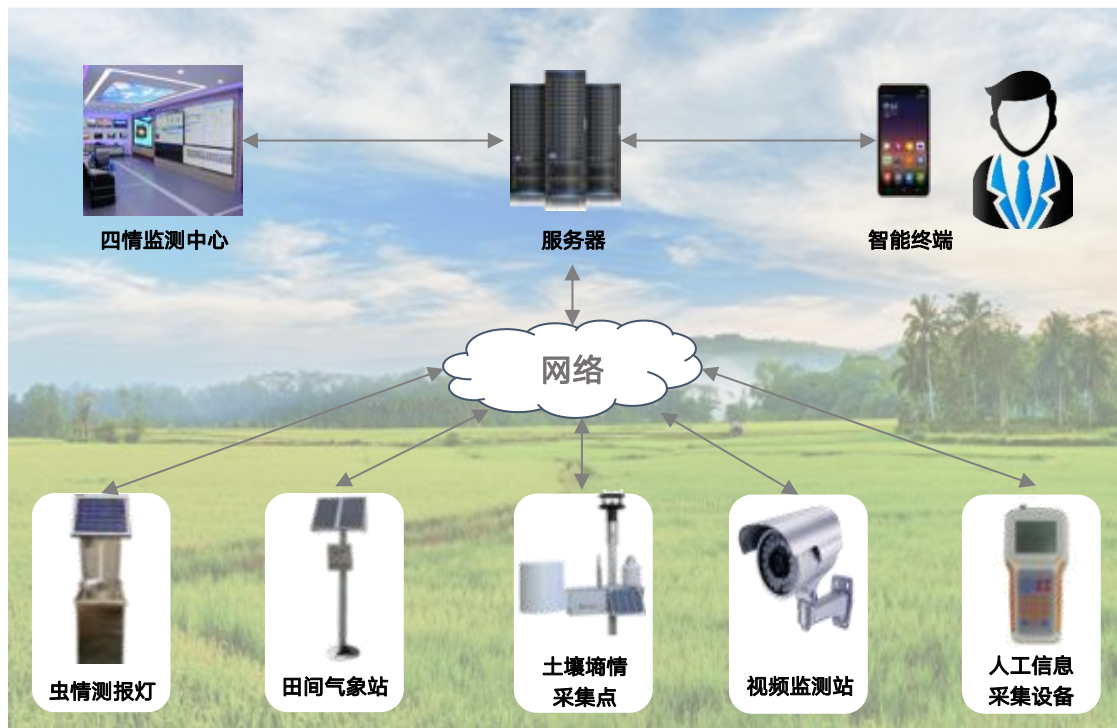
农林“四情”检测智能化解决方案架构
