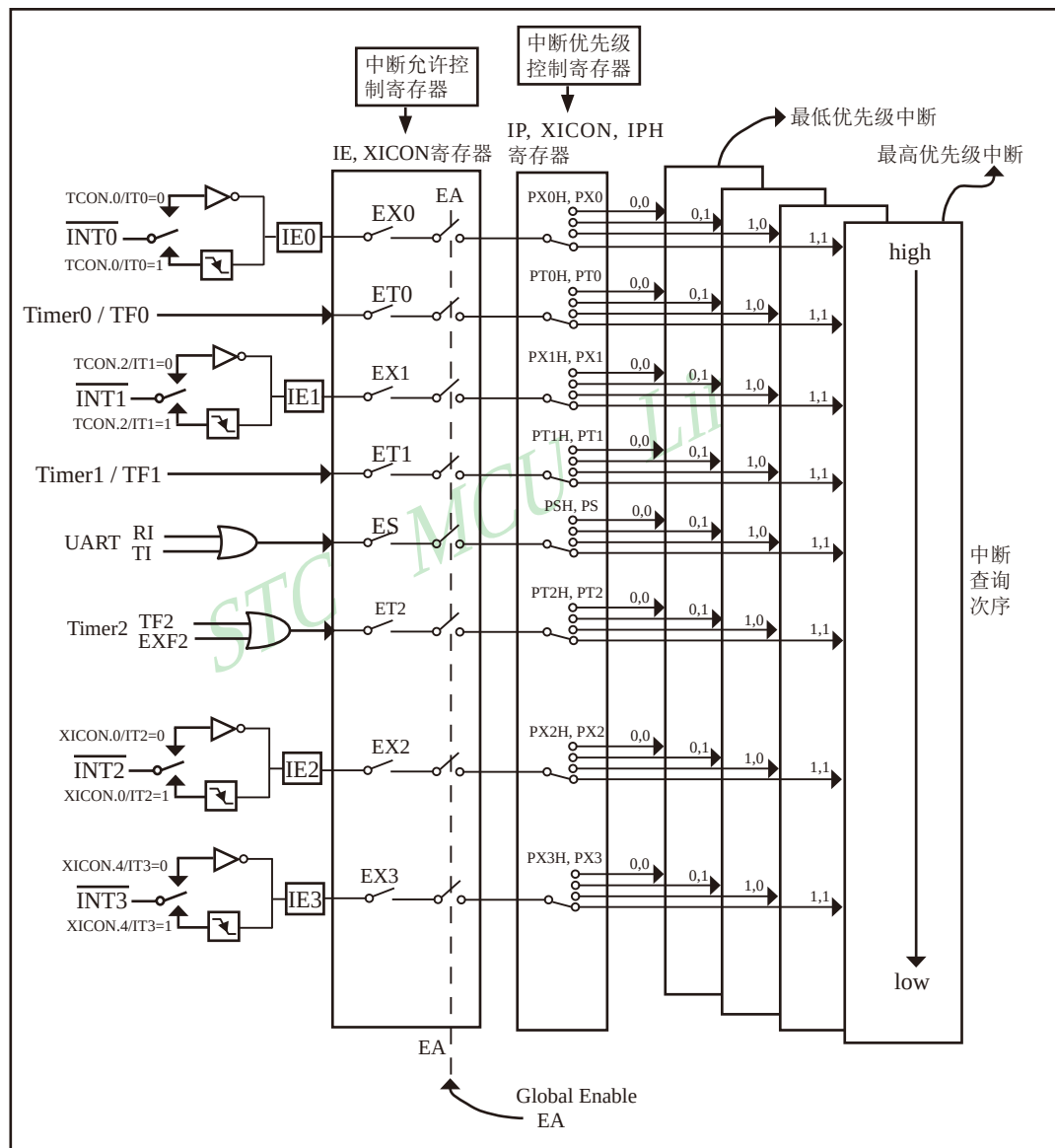
图6-1 STC89C52系列中断系统结构图
