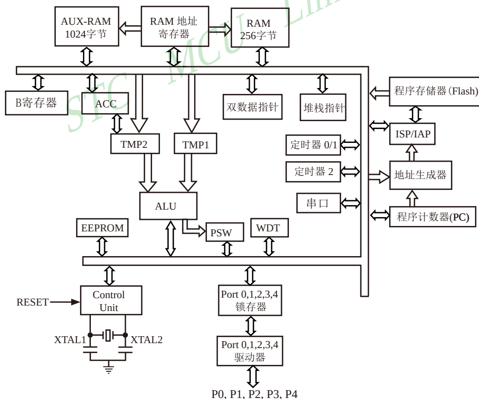
STC89C52系列内部结构框图
