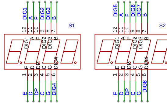
共阴数码管
