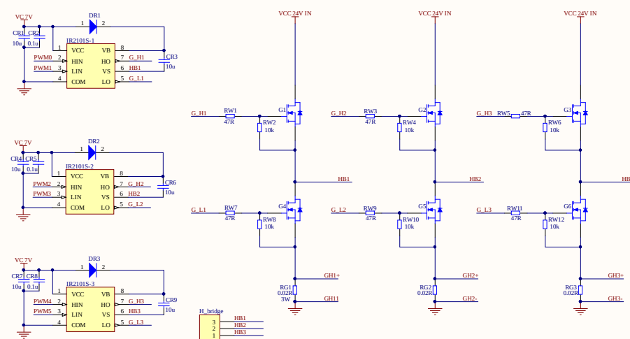
三相裂变桥及驱动
