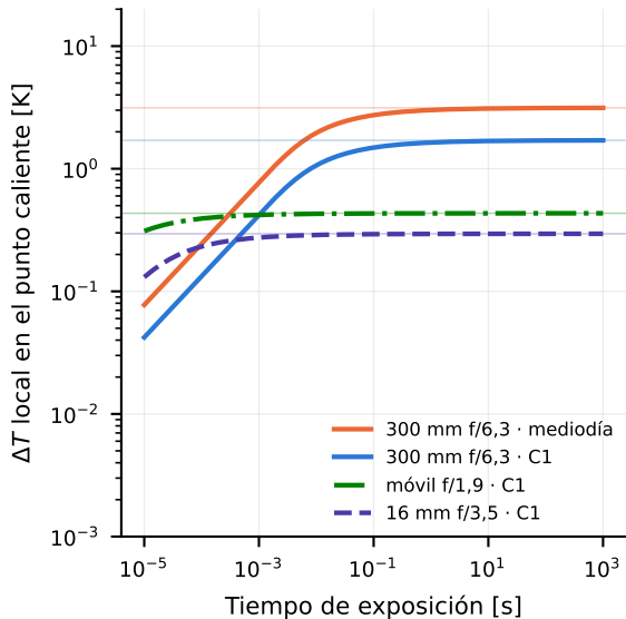
Constricción local (Carslaw & Jaeger)
