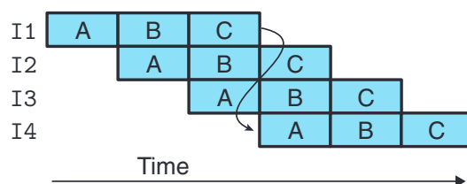
(d) Pipeline diagram
