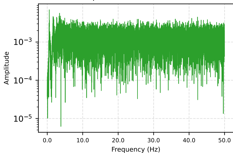
DYN1-9Y — Spectrum
