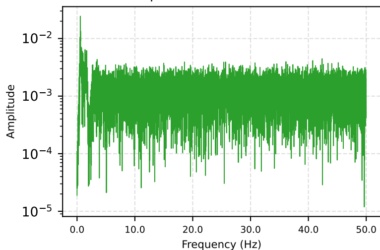
DYN1-2X — Spectrum
