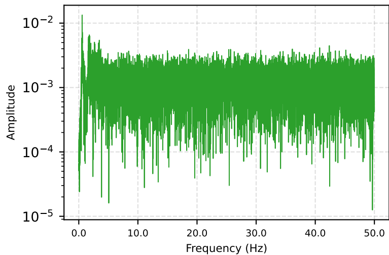
DYN1-18X — Spectrum
