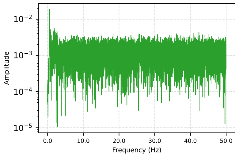
DYN1-16Y — Spectrum
