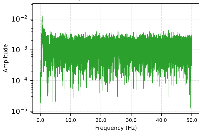
DYN1-3Y — Spectrum
