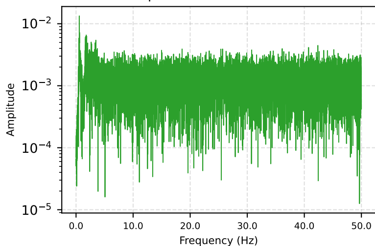
DYN1-8X — Spectrum
