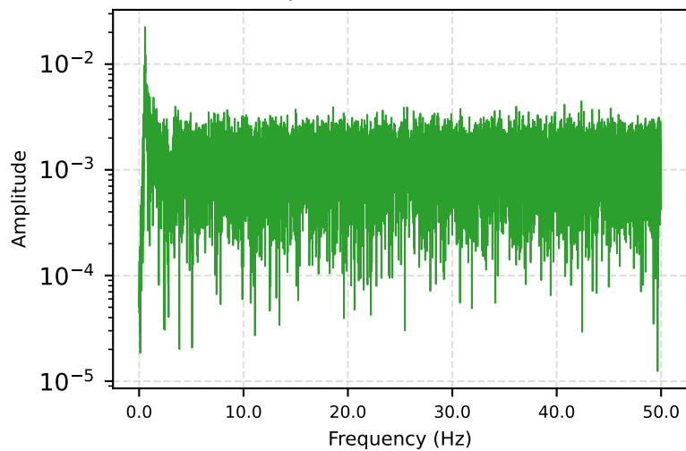
DYN1-14Y — Spectrum
