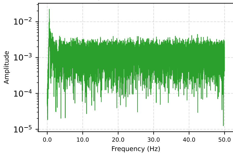
DYN1-13Y — Spectrum
