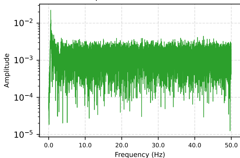
DYN1-4Y — Spectrum
