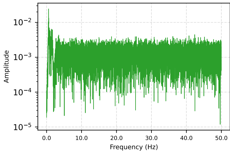
DYN1-12X — Spectrum
