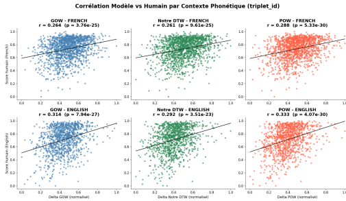
Fig. 5. Corrélation modèle-humain par type de triplets (contexte phonétique global).
