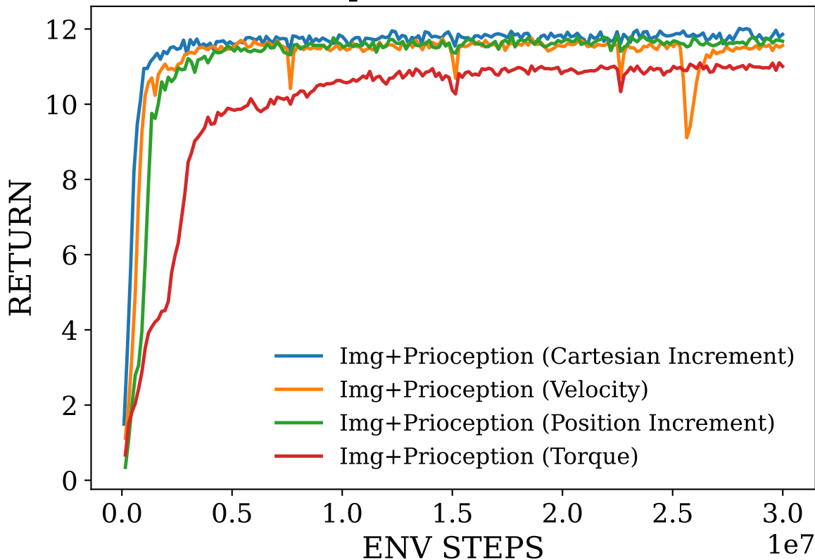
Episodic Return
