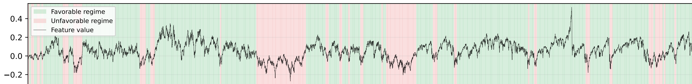
sortino 63d
