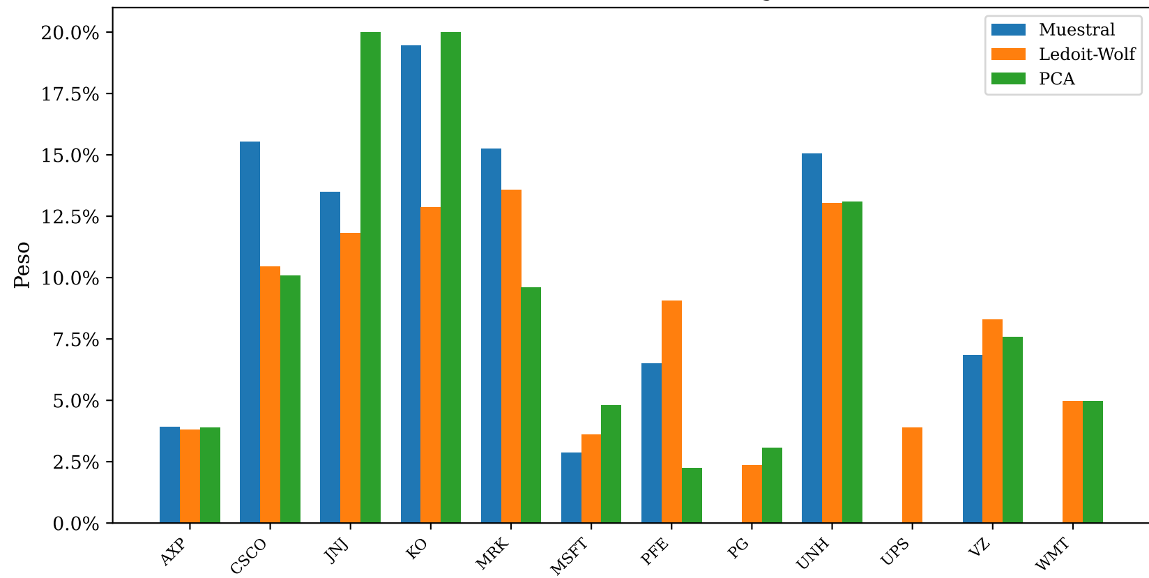
Pesos de la cartera de mínima varianza según estimador de \Sigma
