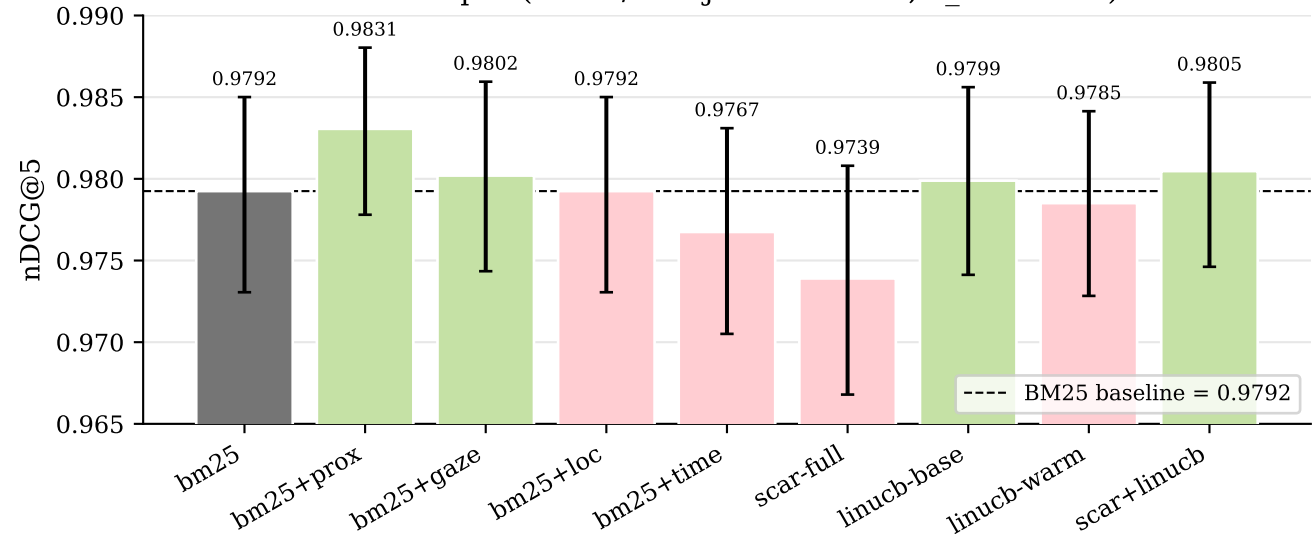
Real corpus (vercel/next.js Discussions, n_obs=1000)
