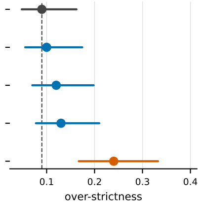
GPT-OSS 20B
