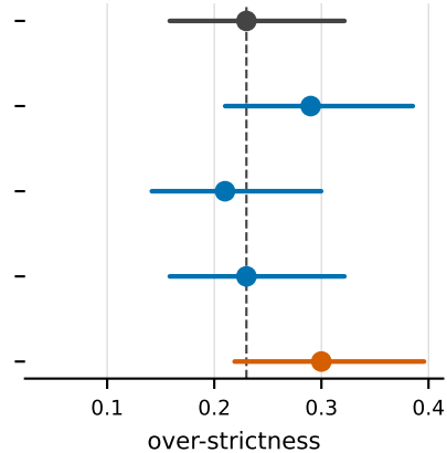
Gemma 3 27B
