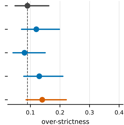
Llama 3.3 70B
