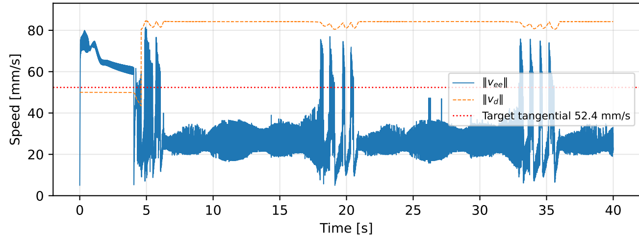
EE Speed: Desired vs. Actual
