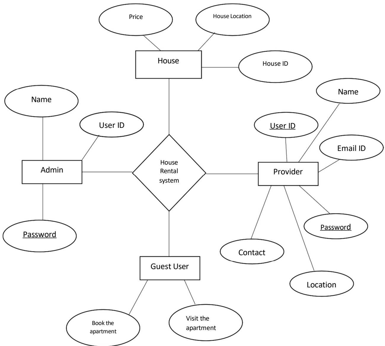
Fig 3.8.1: ER diagram
