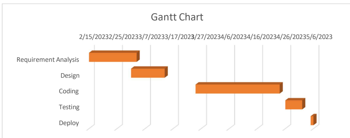
Fig 3.5.1.2: Gantt chart
