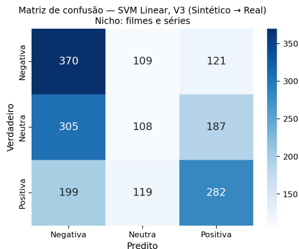
Figura 2. Matriz de confusão do SVM Linear em V3 (Sintético → Real, filmes e séries, 600 frases por classe no teste). A classe Neutra é a mais sacrificada e há transbordamento entre Positiva e Negativa.
