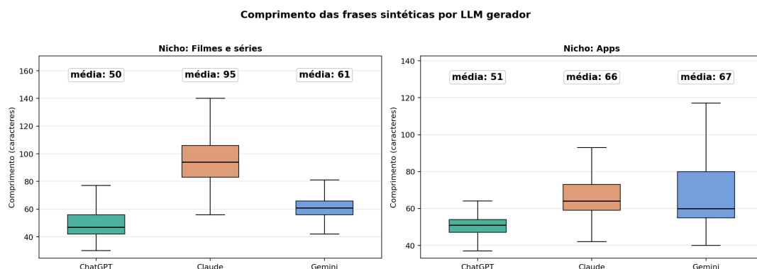
Figura 1. Diagrama de caixa ( boxplot ) do comprimento das frases sintéticas por LLM gerador em cada nicho.
