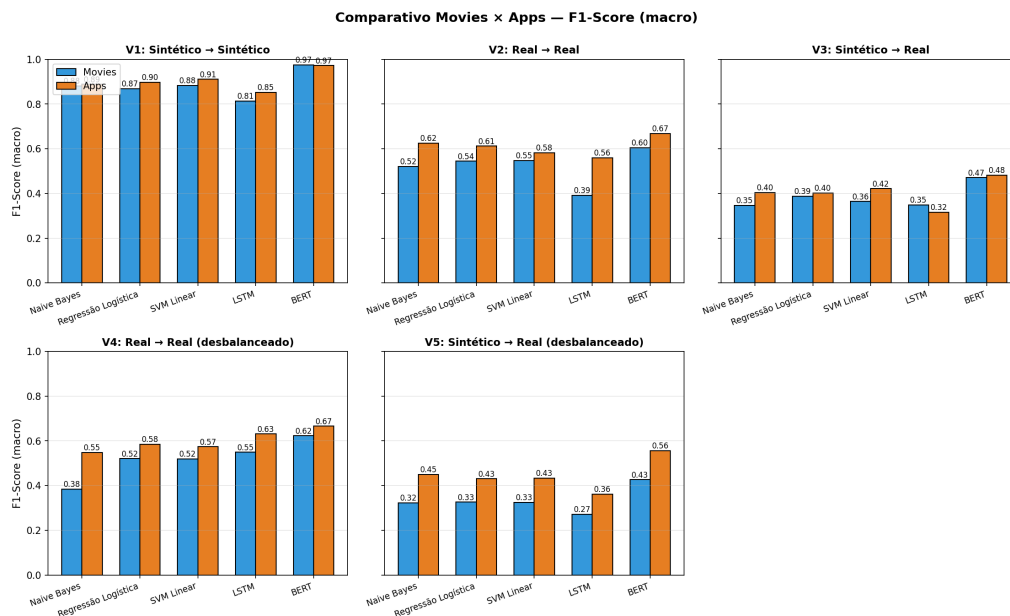
Figura 4. F1-Score macro nas cinco visões para os dois nichos. A diferença em relação ao F1 weighted nas visões V4 e V5 expõe o viés de classe majoritária.
