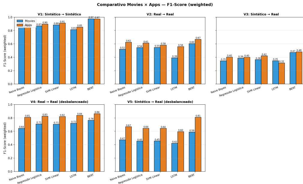
Figura 3. F1-Score weighted nas cinco visões para os dois nichos (Filmes e séries / Apps).
