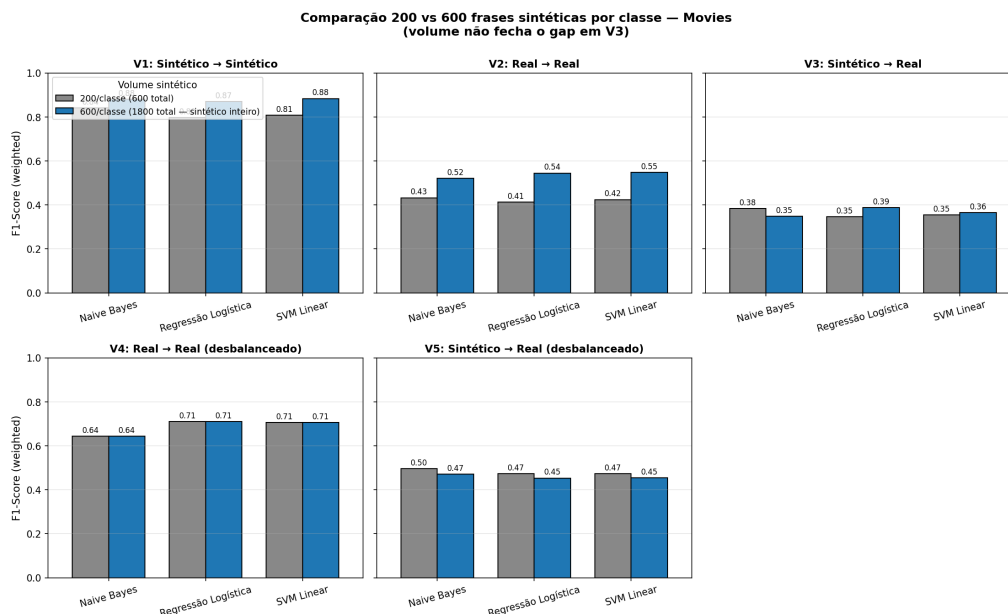
Figura 5. Comparação do desempenho em filmes e séries com 200 vs 600 frases sintéticas por classe. Volume não fecha o gap em V3.
