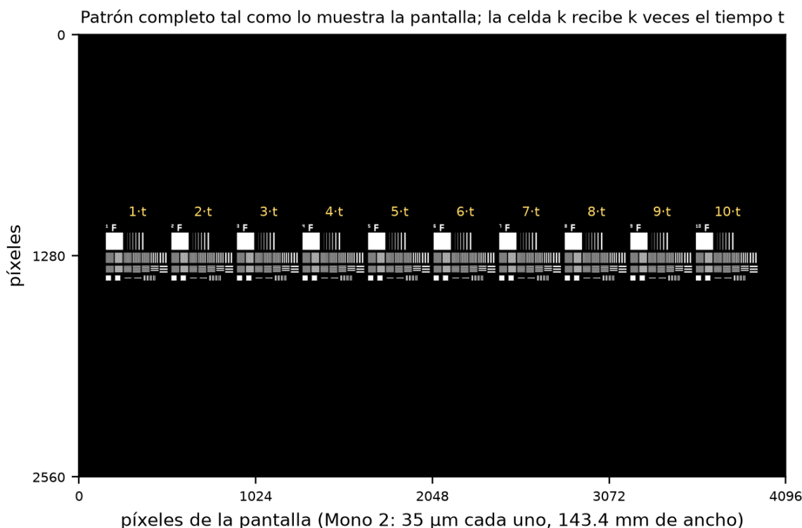
Figura 2. El patrón completo generado para la Mono 2 (4096 × 2560 px); en otros modelos cambia la resolución y la app reacomoda las celdas, pero el contenido es el mismo. El archivo tiene diez capas; la celda k aparece en las primeras k capas, así que recibe k veces el tiempo t.
