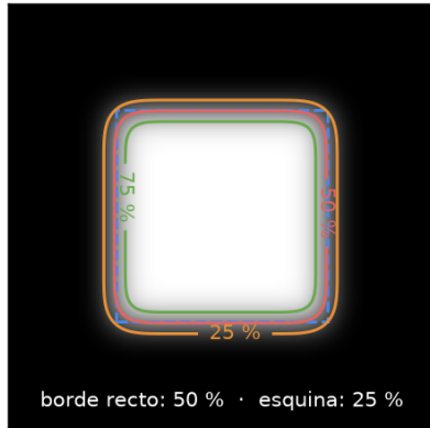
Dosis relativa que recibe la resina (línea azul punteada: diseño)
