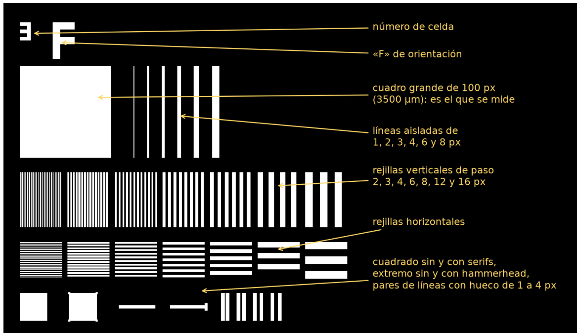
Figura 3. Contenido de una celda. Las medidas en micras corresponden a la Mono 2 (35 μm por píxel); en otros modelos el cuadro grande sigue siendo de 100 píxeles, es decir 100 veces el tamaño de píxel. Para el ajuste de \sigma y D_0 solo se mide el cuadro; el resto sirve para comprobar el resultado.
