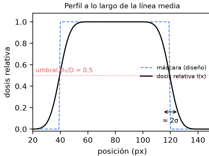
Figura 6. Dosis relativa alrededor de un cuadrado expuesto. La resina revela donde la dosis supera D_0 , es decir donde I \geq D_0/D .
