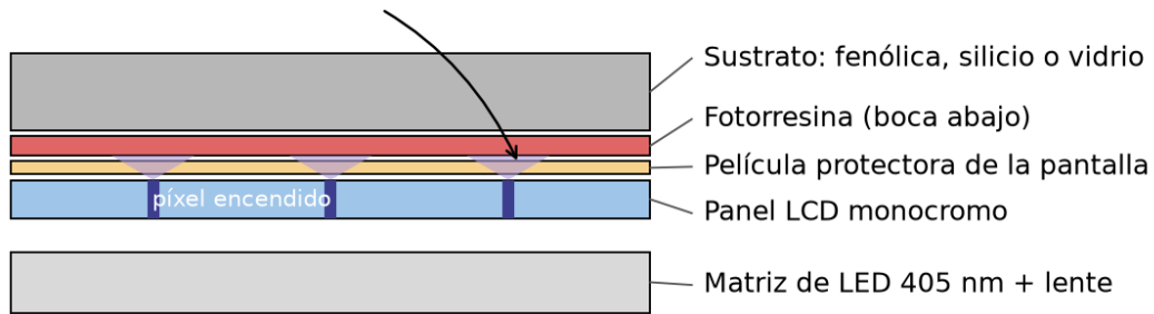
Figura 1. Corte del montaje. La resina va en contacto con la película protectora de la pantalla. La luz de cada píxel sale divergente, así que cualquier separación se convierte en desenfoque.
