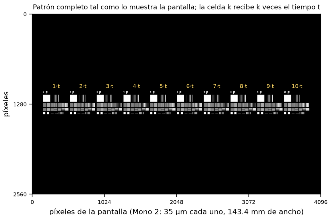
Figura 2. El patrón completo generado para la Mono 2 (4096 × 2560 px); en otros modelos cambia la resolución y la app reajusta las celdas, pero el contenido es el mismo. El archivo tiene diez capas; la celda k aparece en las primeras k capas, así que recibe k veces el tiempo t.
