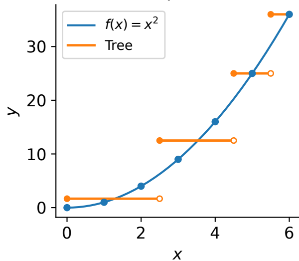
Depth 2
