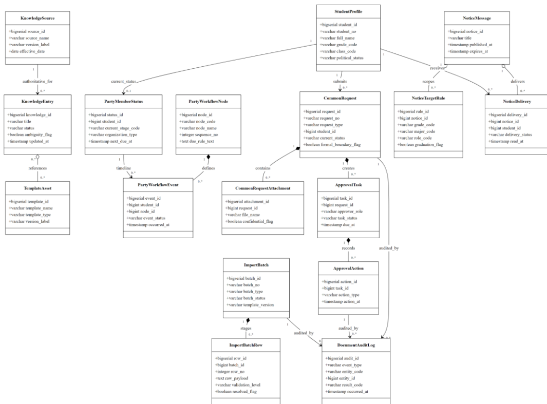
图 3-3 核心业务分析类图
