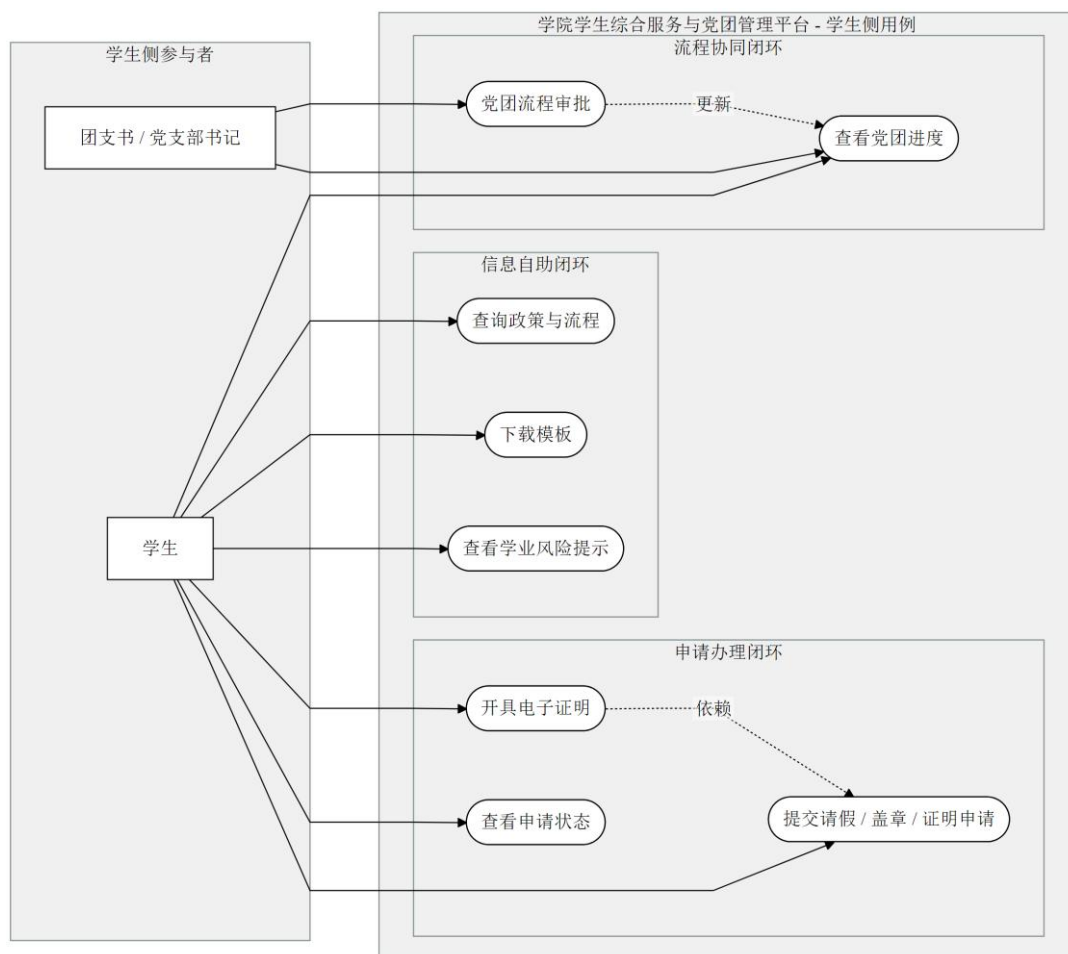
图 3-1 学生侧全局用例图
