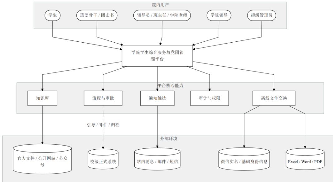
图 2-1 软件产品与外部环境关系图
