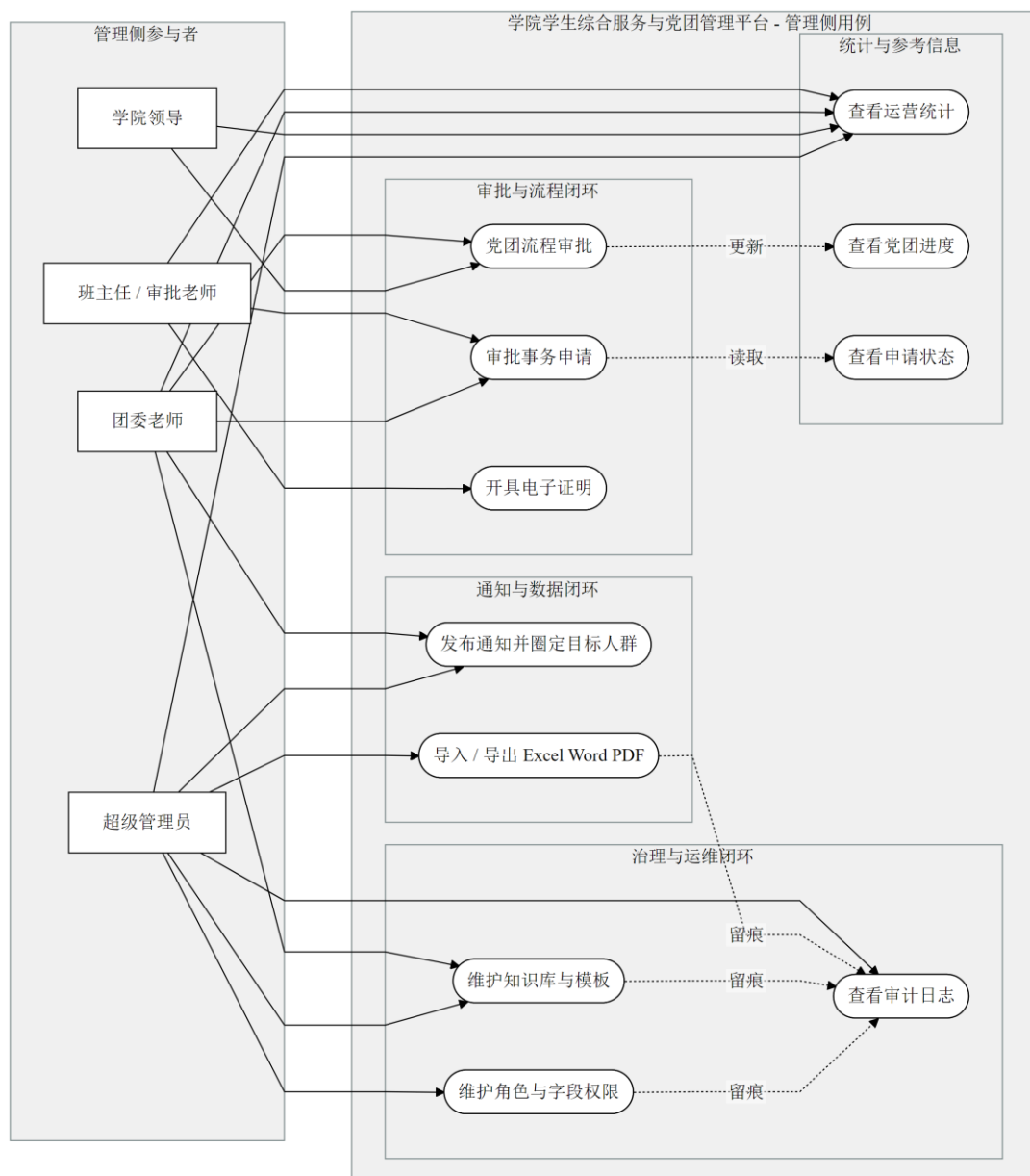
图 3-2 管理侧全局用例图
