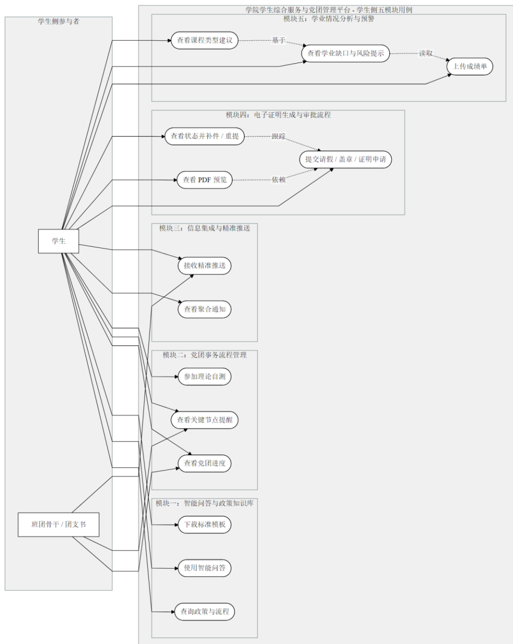
图 3-1 学生侧五模块用例图
