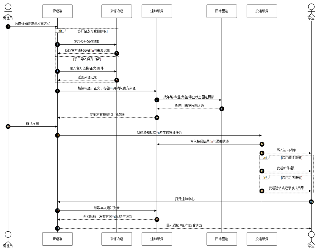
图 3-6 官方信息汇聚与精准推送时序图
