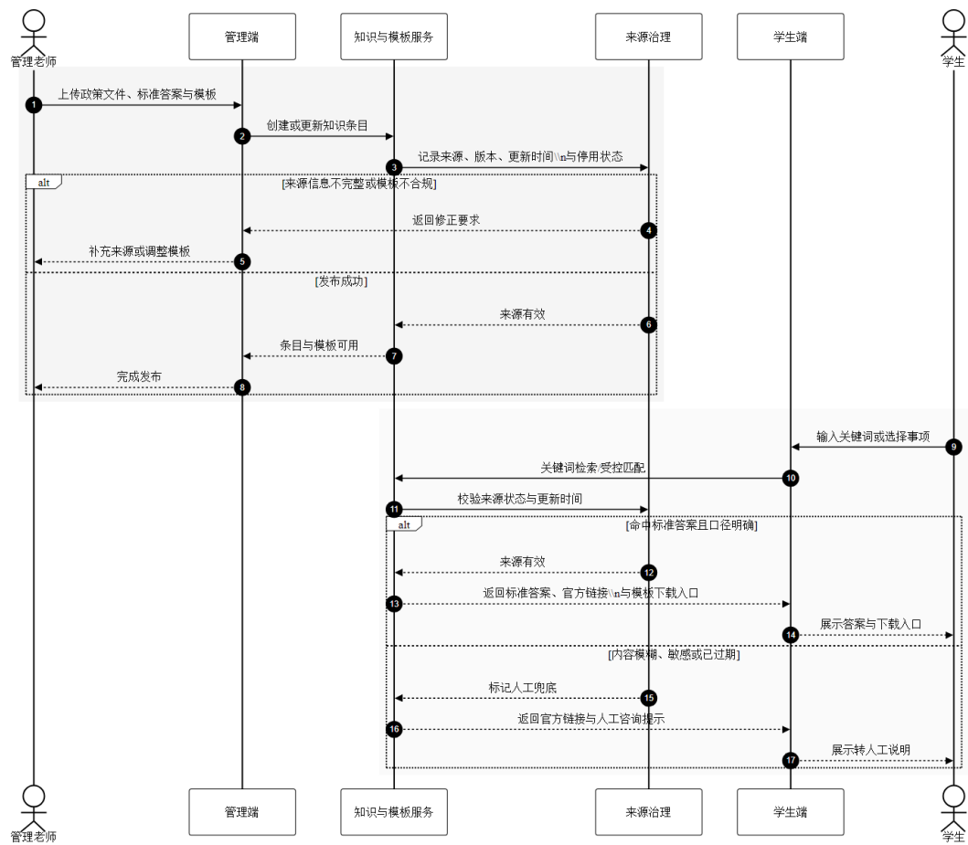
图 3-4 知识问答与模板下载时序图
