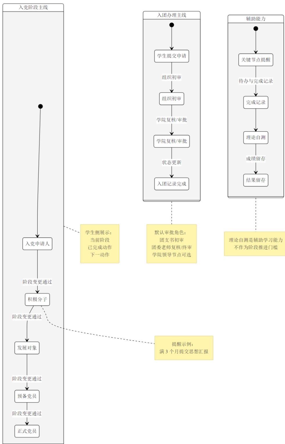
图 3-5 党团事务流程状态图
