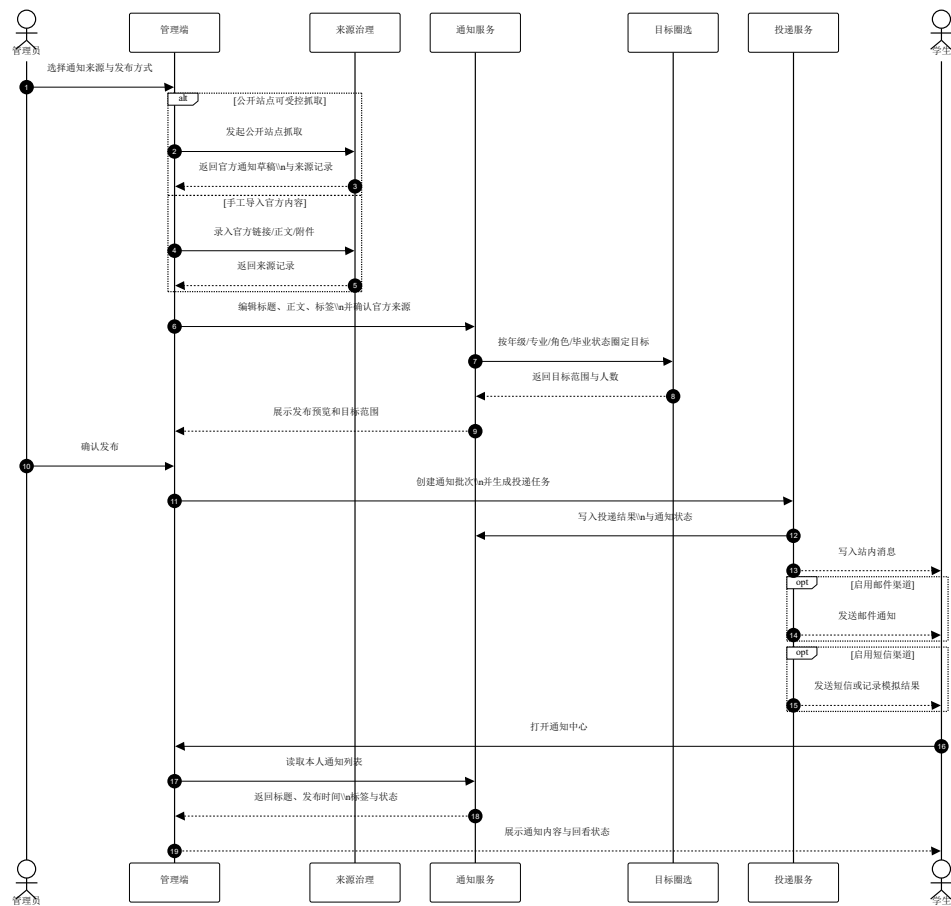
图 3-7 官方信息汇聚与精准推送时序图
