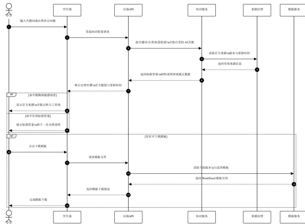
图 3-5 知识问答与模板下载时序图
