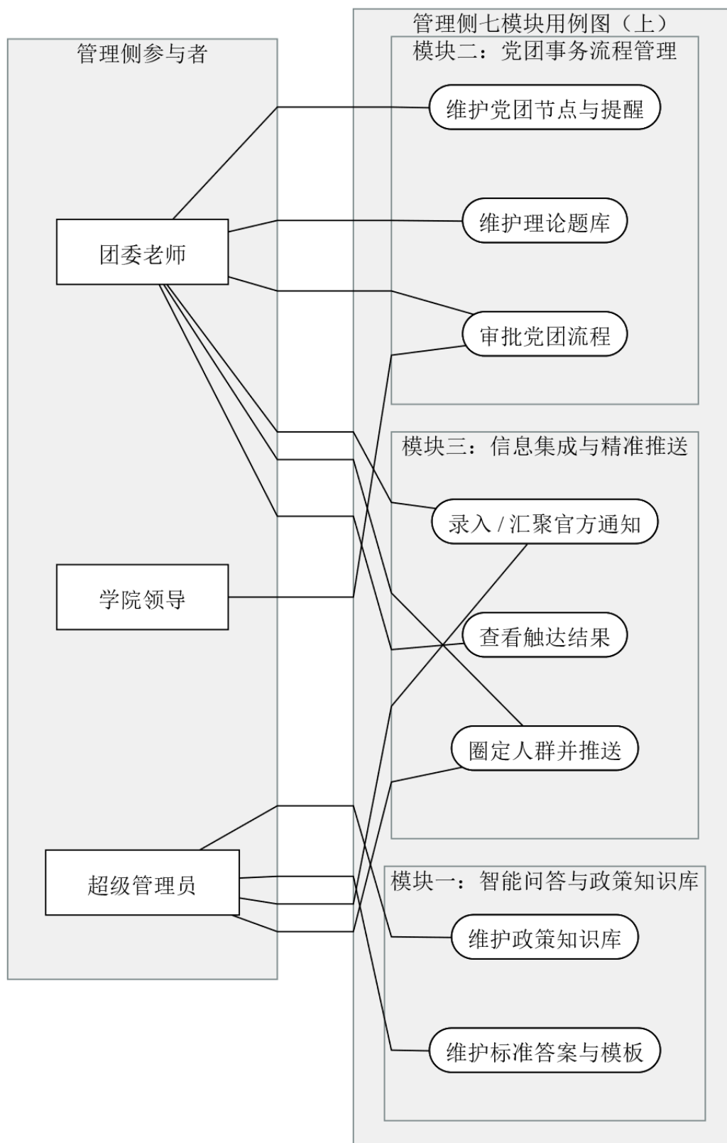
图 3-2（a）管理侧七模块用例图（知识库、党团事务与通知推送）
