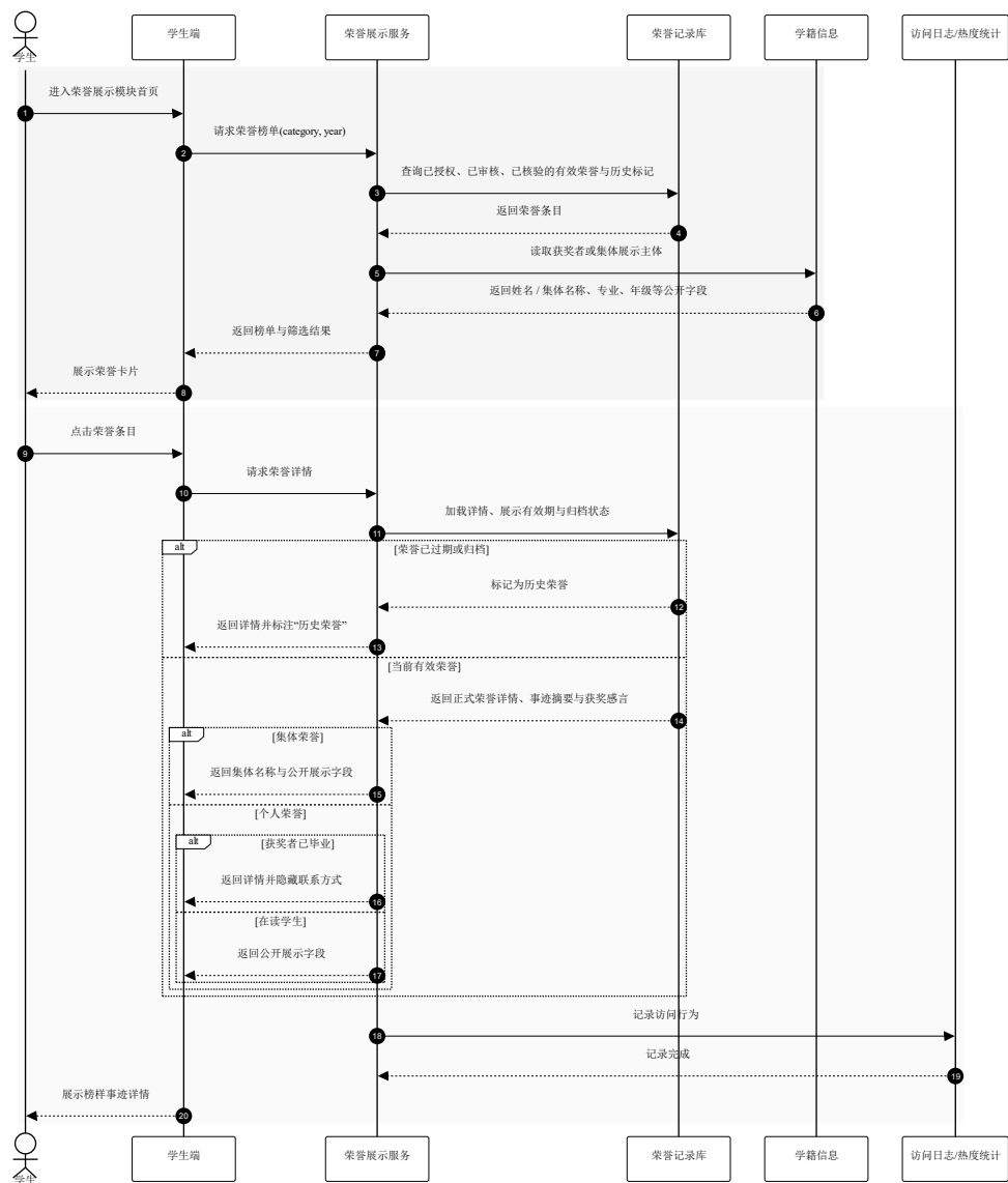
图 3-10 荣誉榜单浏览与详情查看时序图
