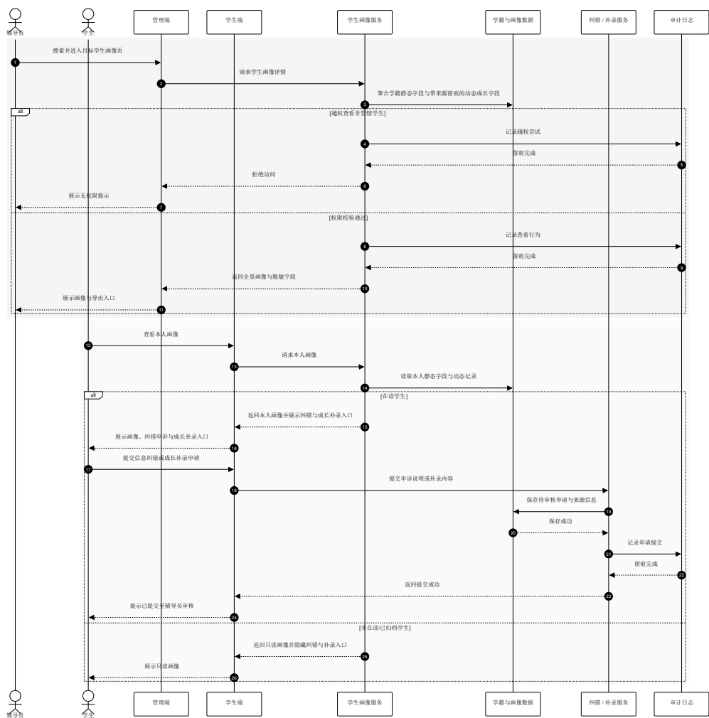
图 3-11 学生画像查看与纠错 / 成长补录时序图
