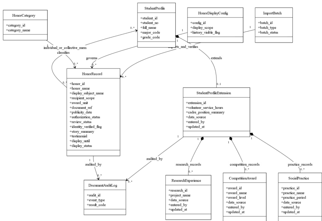
图 3-4 奖励荣誉与学生画像扩展类图
