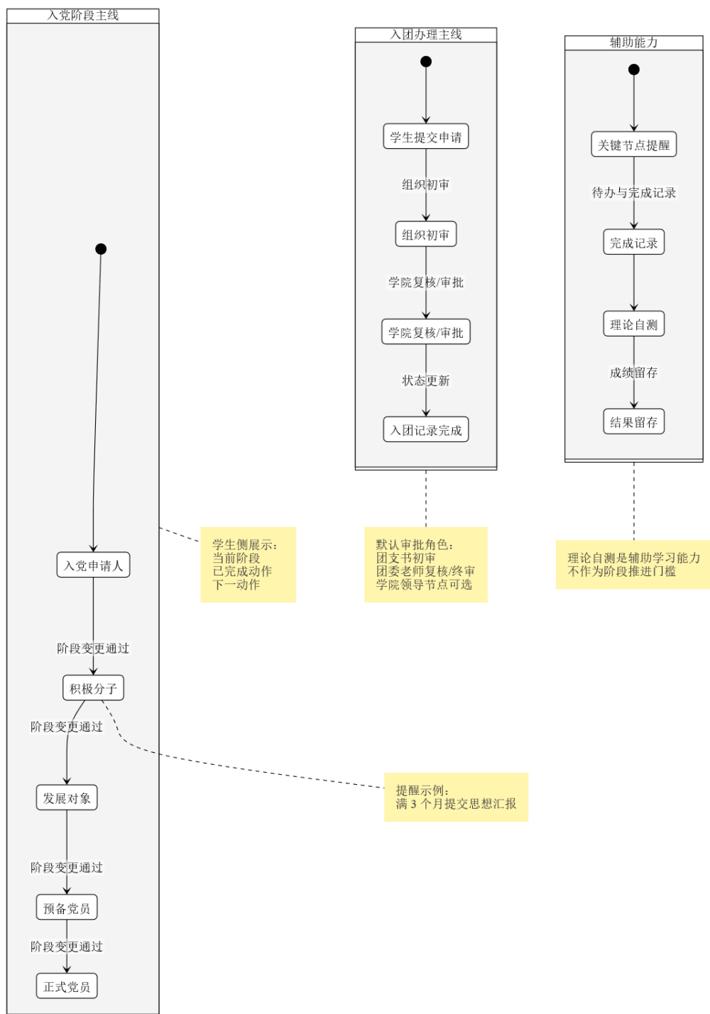
图 3-6 党团事务流程状态图
