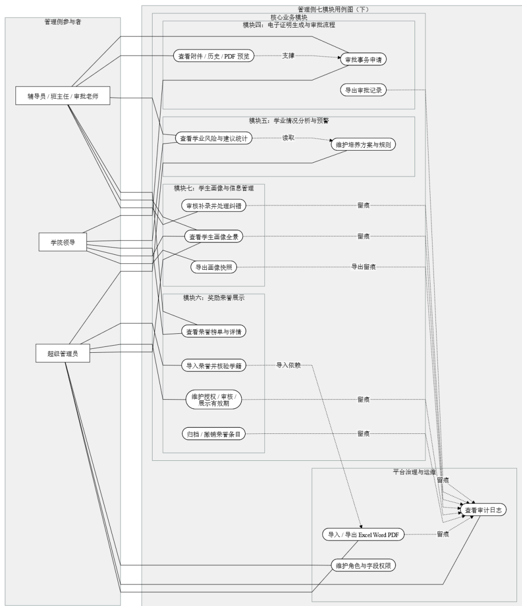
图 3-2（b）管理侧七模块用例图（证明审批、预警分析、荣誉、画像与治理）
