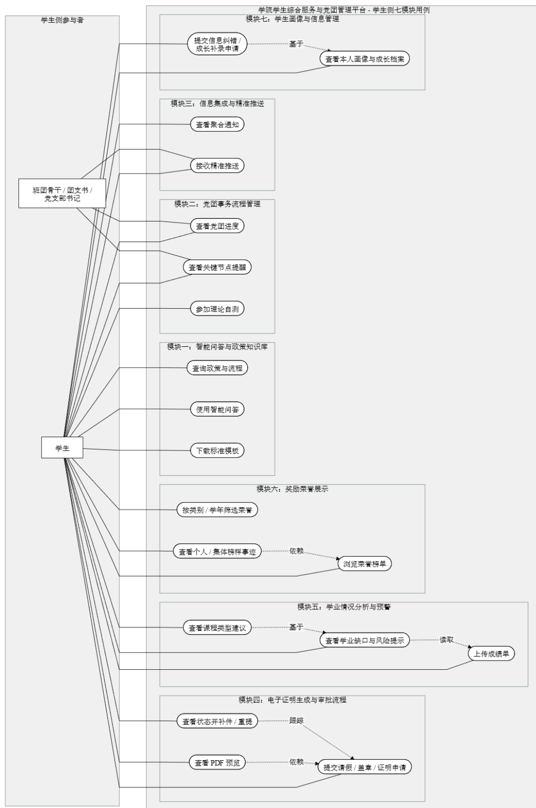
图 3-1 学生侧七模块用例图
