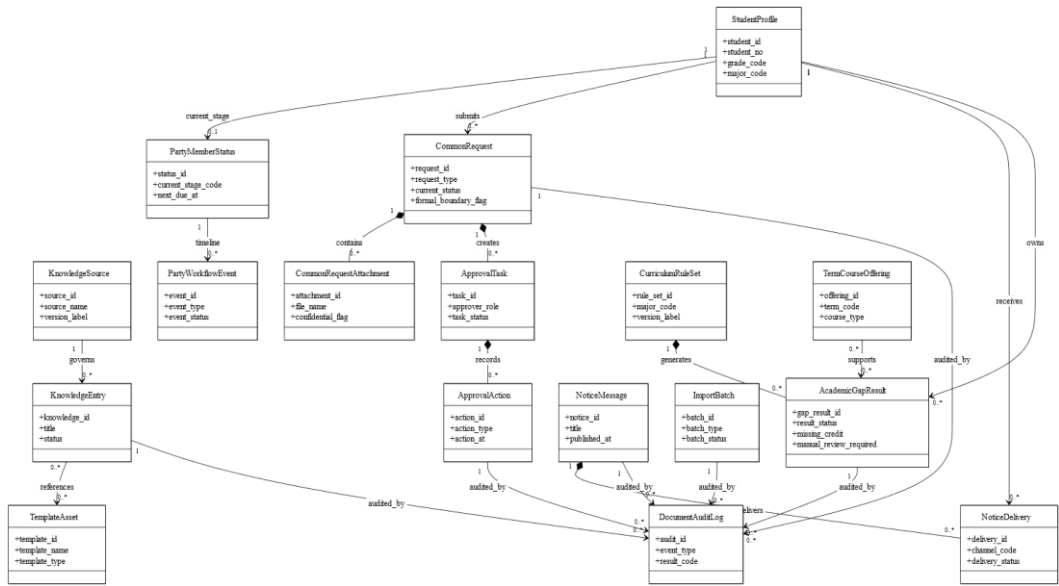
图 3-3 核心业务分析类图
