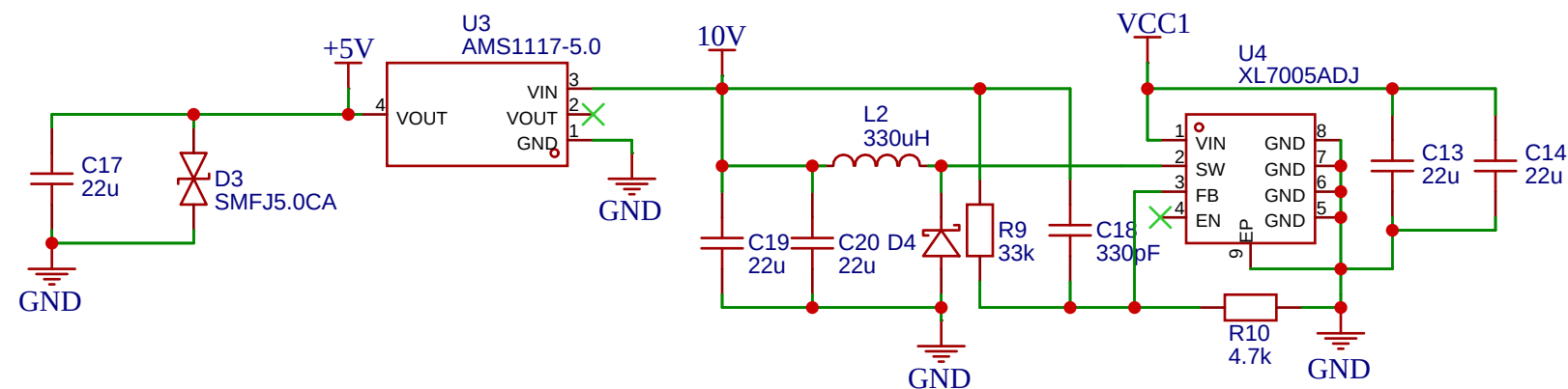
电源部分
