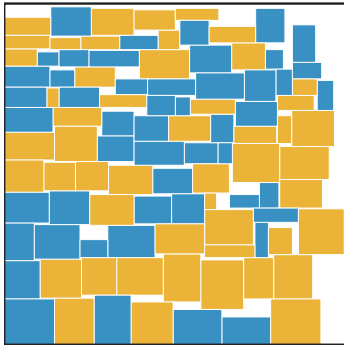
a n100 开发实例, P2-ON 种子 1102 | HPWL 245,513.0
