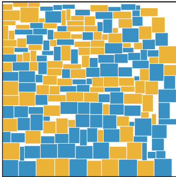
b n200 正式选型, P1 种子 2210 | HPWL 487,309.5
