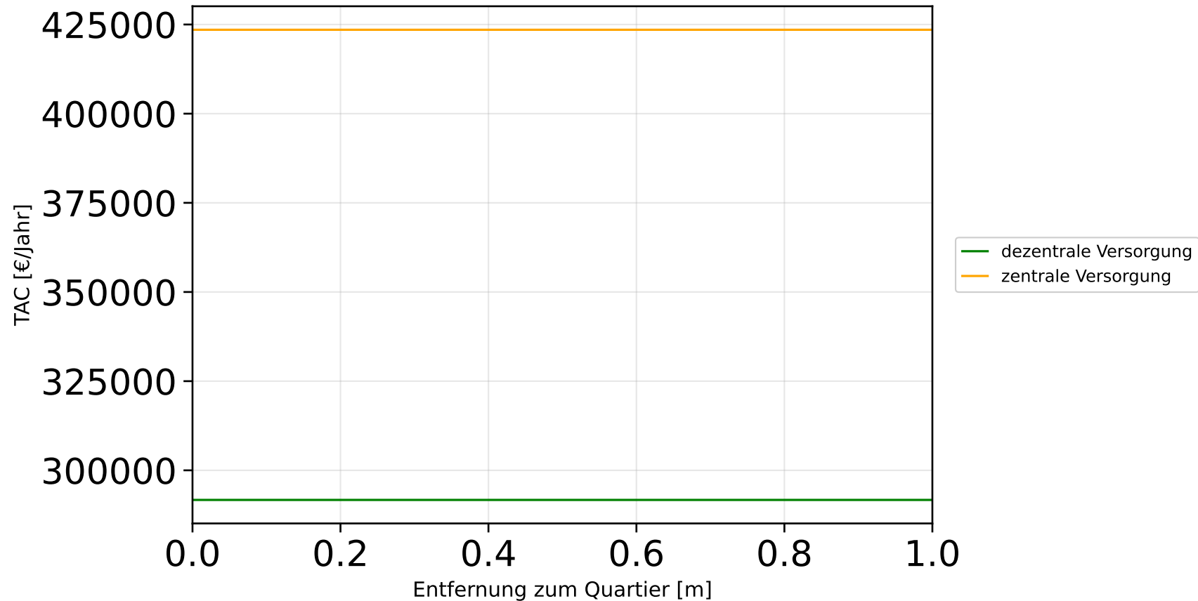
TAC für Milchverarbeitung in Abhängigkeit der Entfernung und Abwärmepreise
