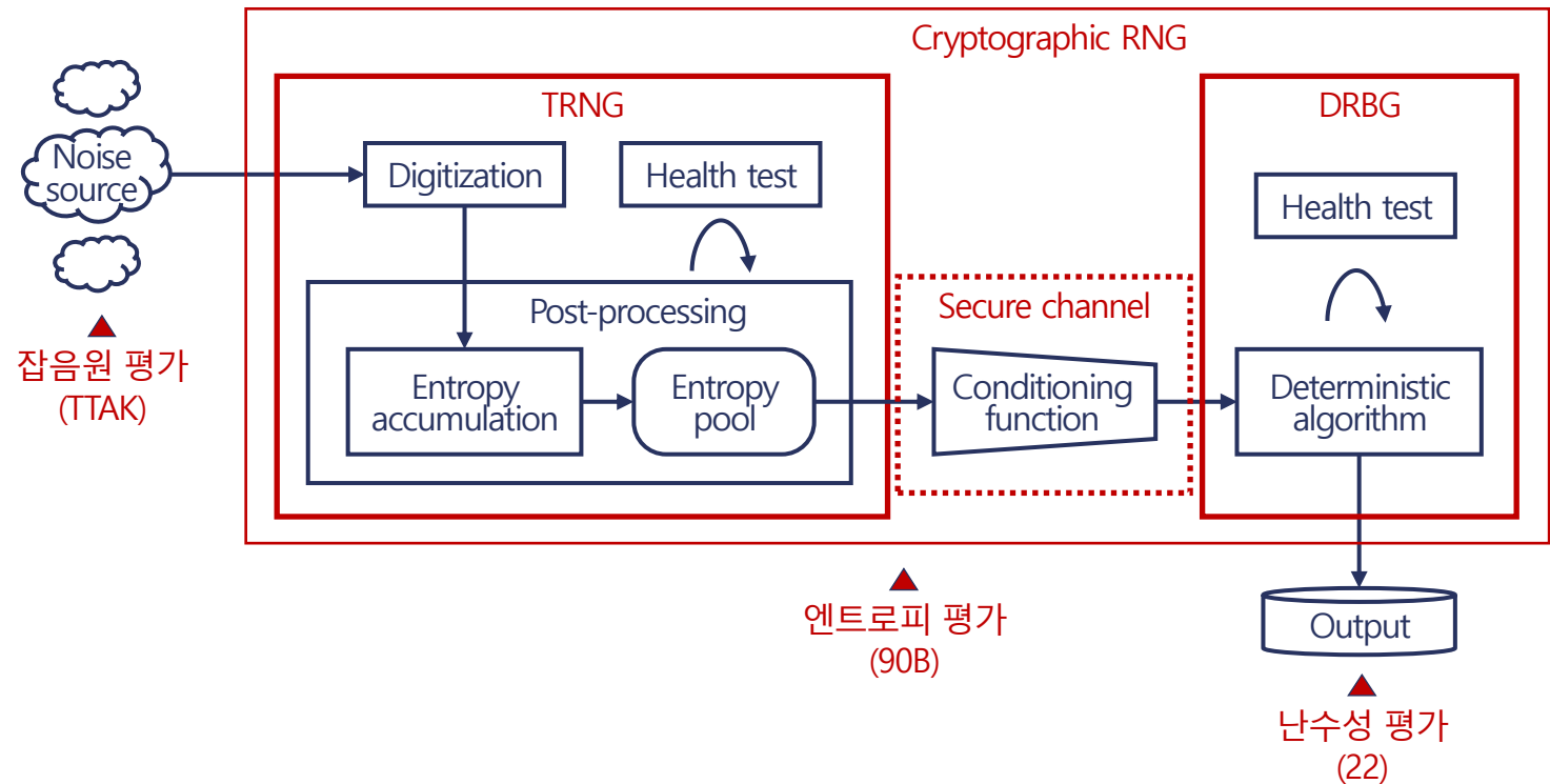
<암호학적 난수발생기의 구조>
