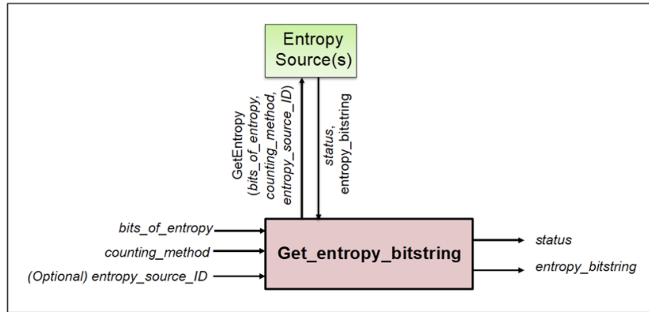
Fig. 10. Get_entropy_bitstring function
