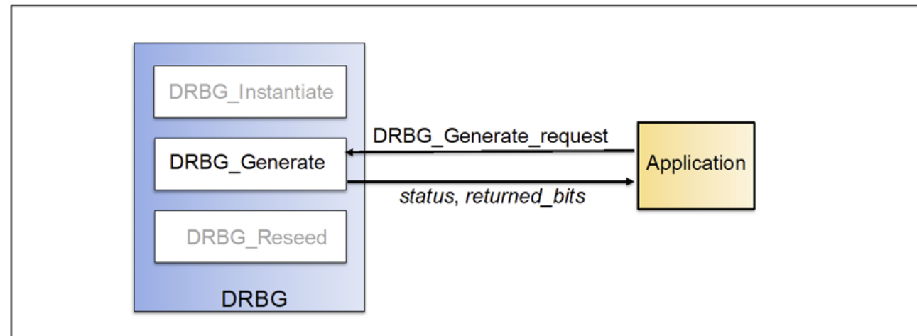
Fig. 7. DRBG_Generate_request
