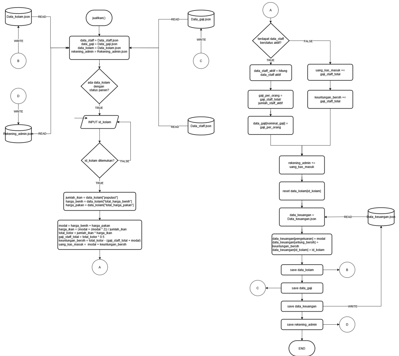
Gambar 3.13 Flowchart Jual Ikan
