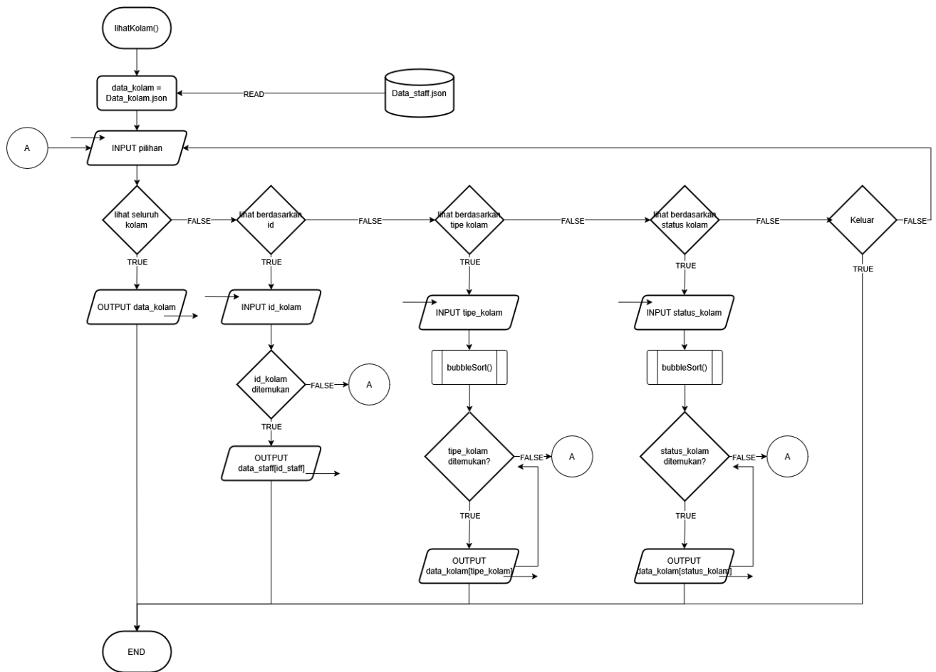
Gambar 3.6 Flowchart Lihat Kolam
