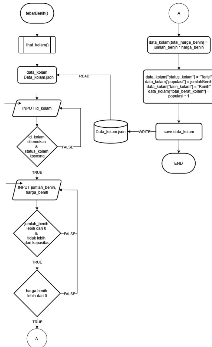
Gambar 3.10 Flowchart Tebar Benih
