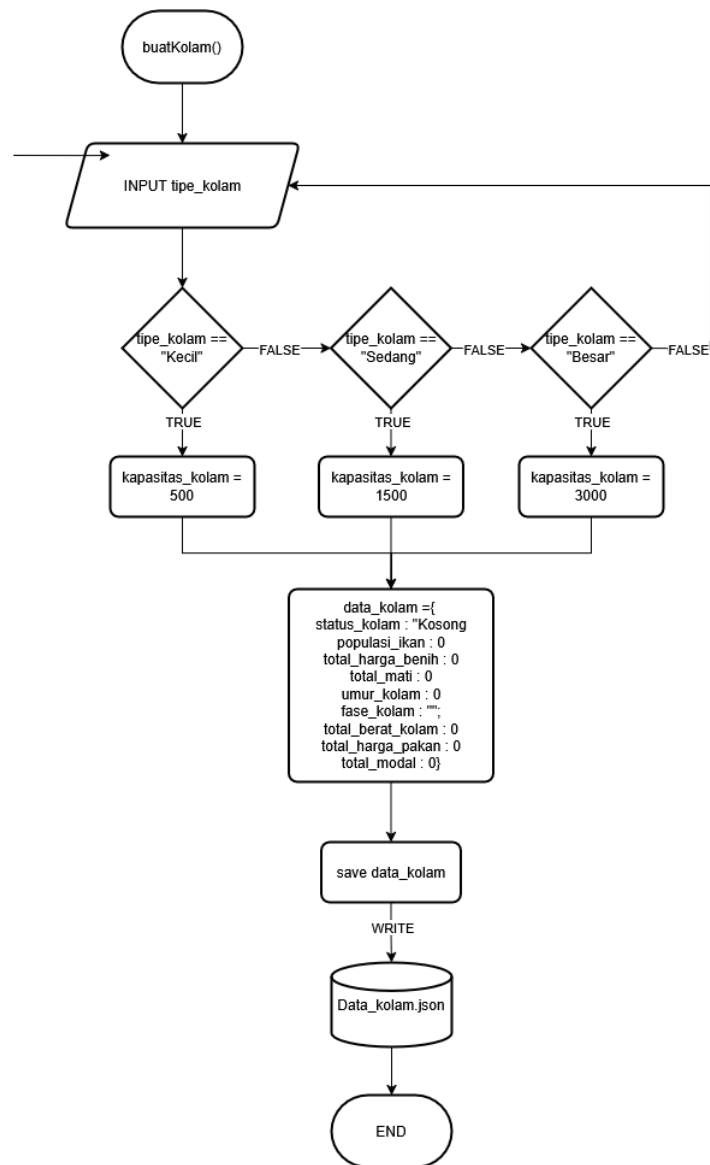
Gambar 3.4 Flowchart Buat Kolam
