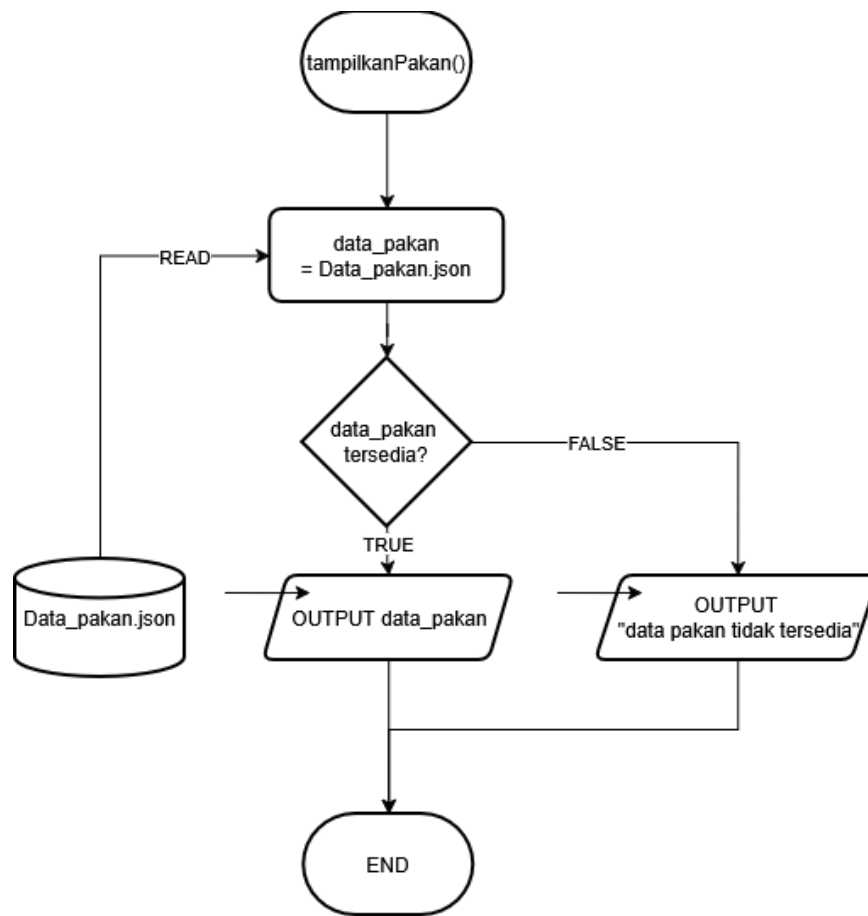
Gambar 3.12 Flowchart Tampilkan Pakan
