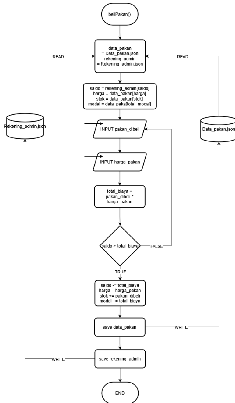
Gambar 3.11 Flowchart Beli Pakan
