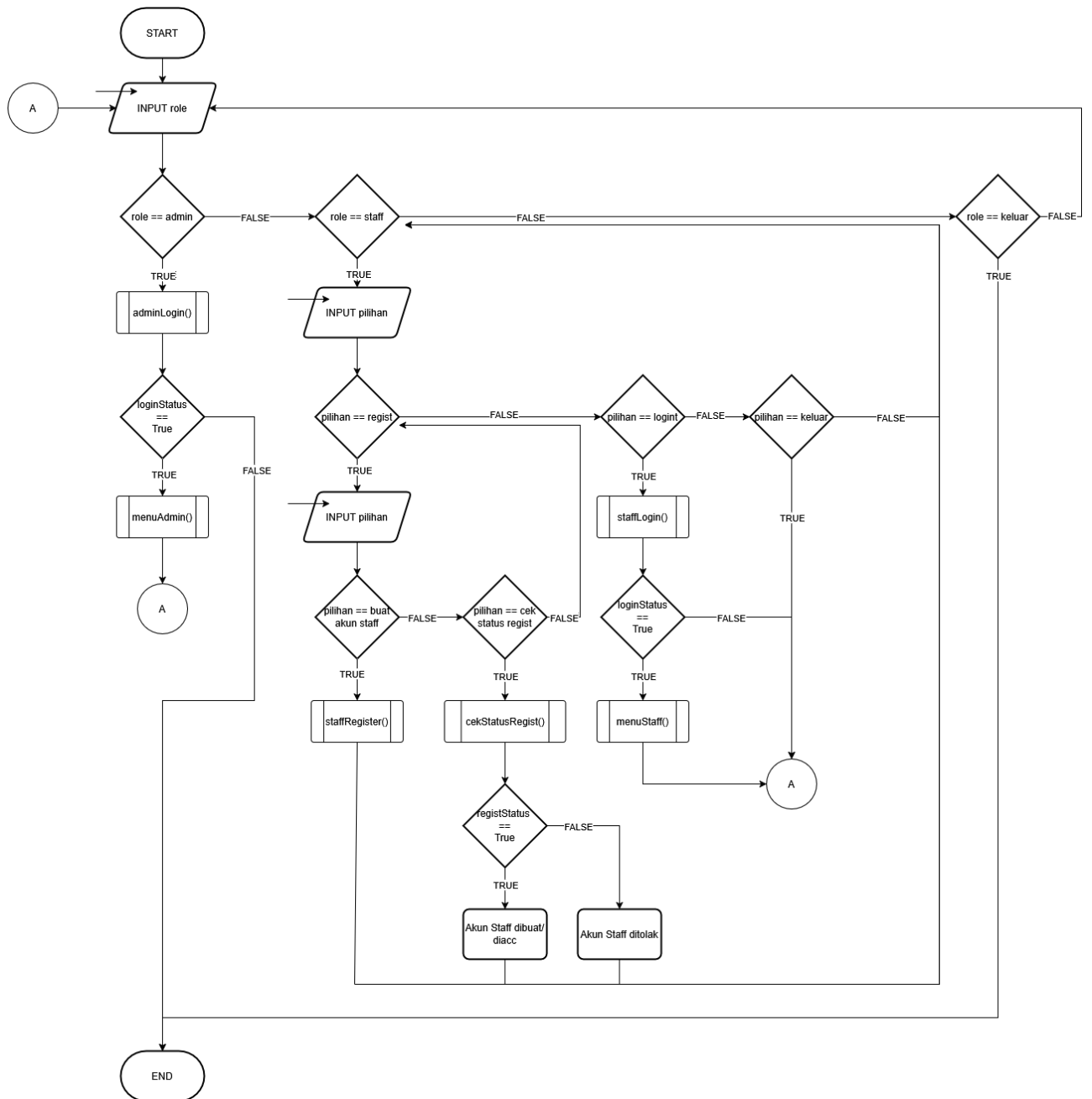
Gambar 3.1 Flowchart Menu Utama
