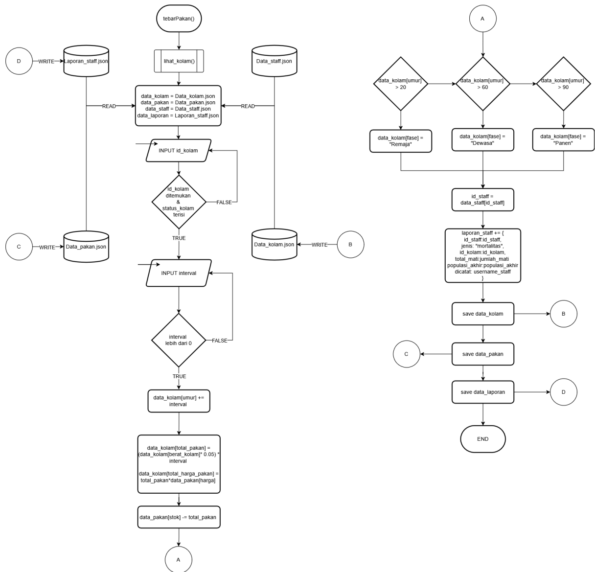
Gambar 3.21 Flowchart Tebar Pakan
