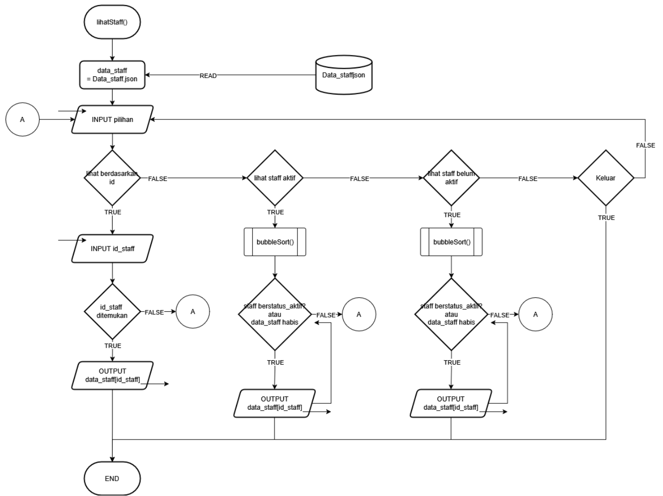
Gambar 3.9 Flowchart Lihat Staff
