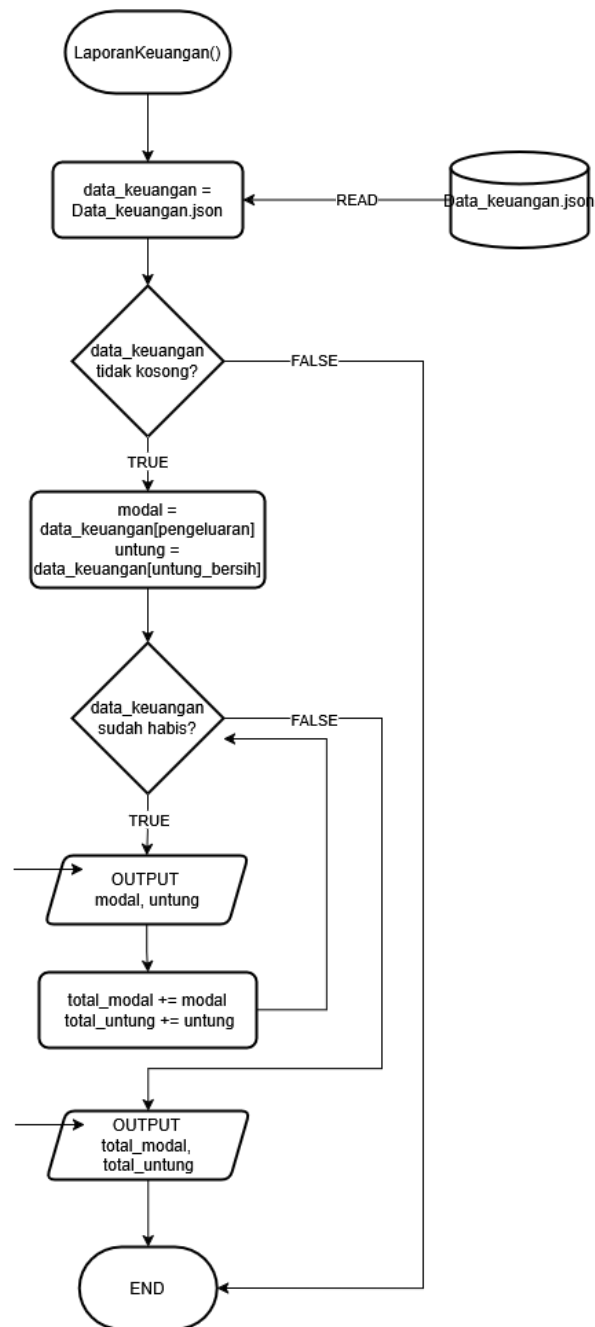
Gambar 3.14 Flowchart Laporan Keuangan
