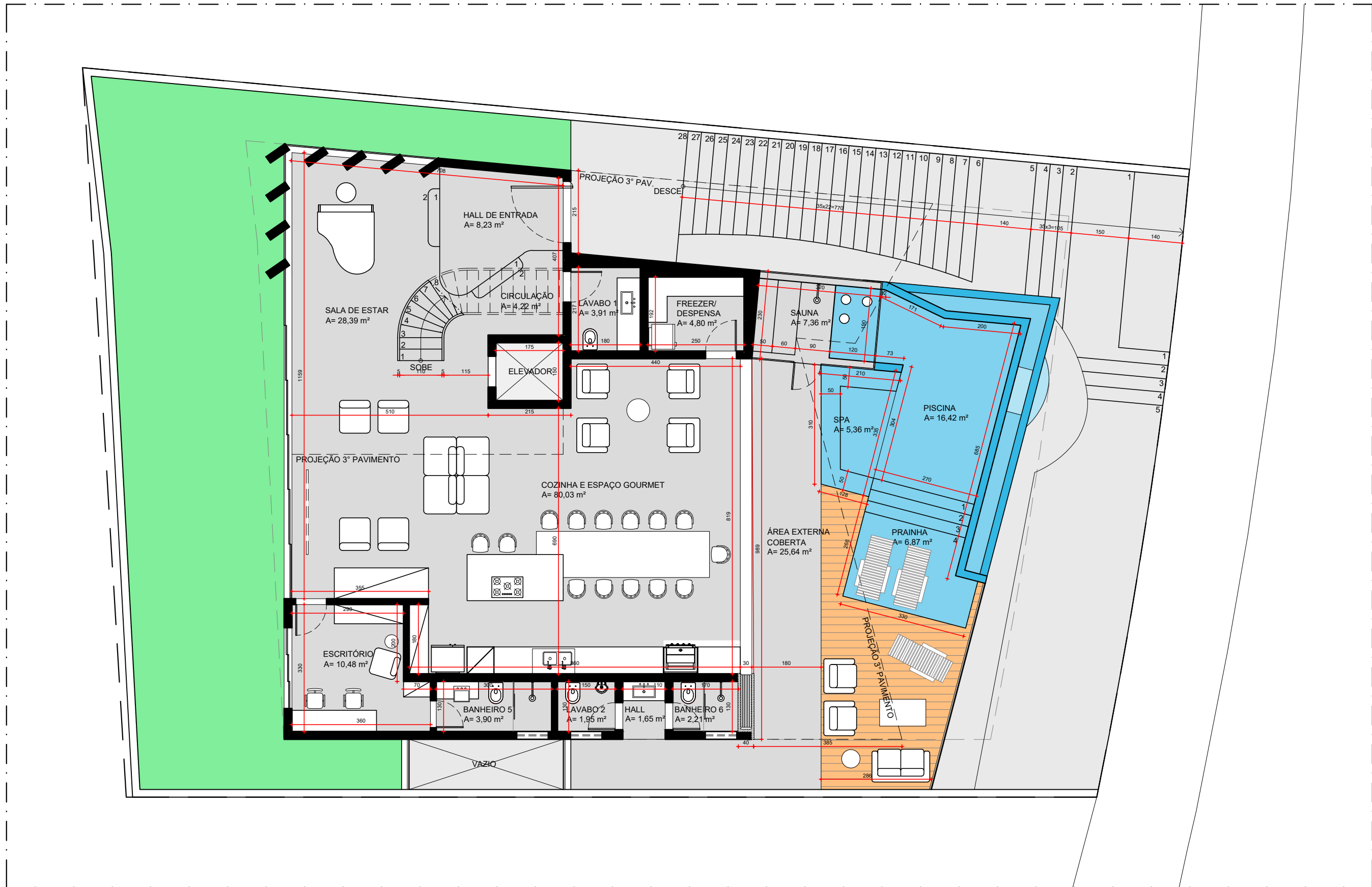
PLANTA 2º PAVIMENTO ESCALA: 1/100 ÁREA EDIFICADA: 223,24 m²
