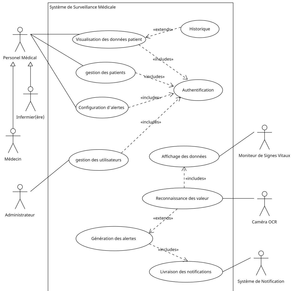
Figure 2.1: Diagramme des cas d'utilisation global
