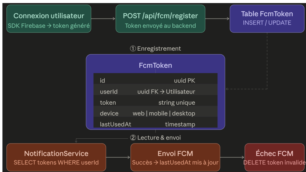
FIGURE 6.4 – Cycle de vie d'un jeton FCM en base de données
