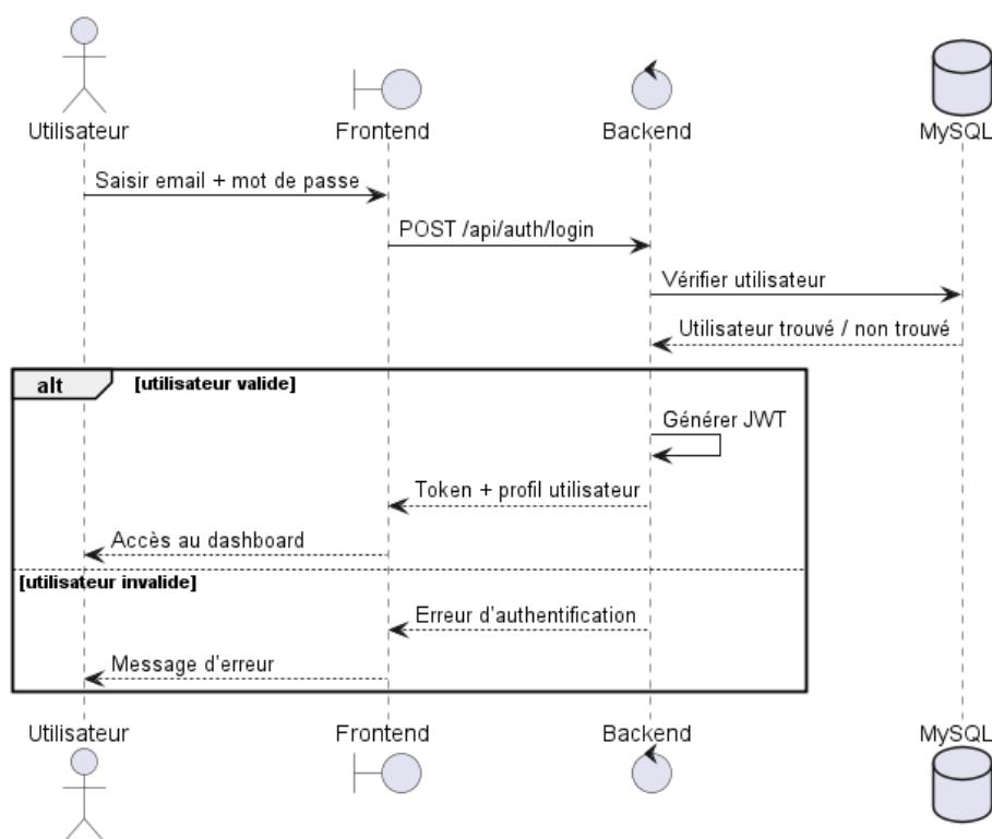
FIGURE 3.5 – Diagramme de séquence d'authentification
