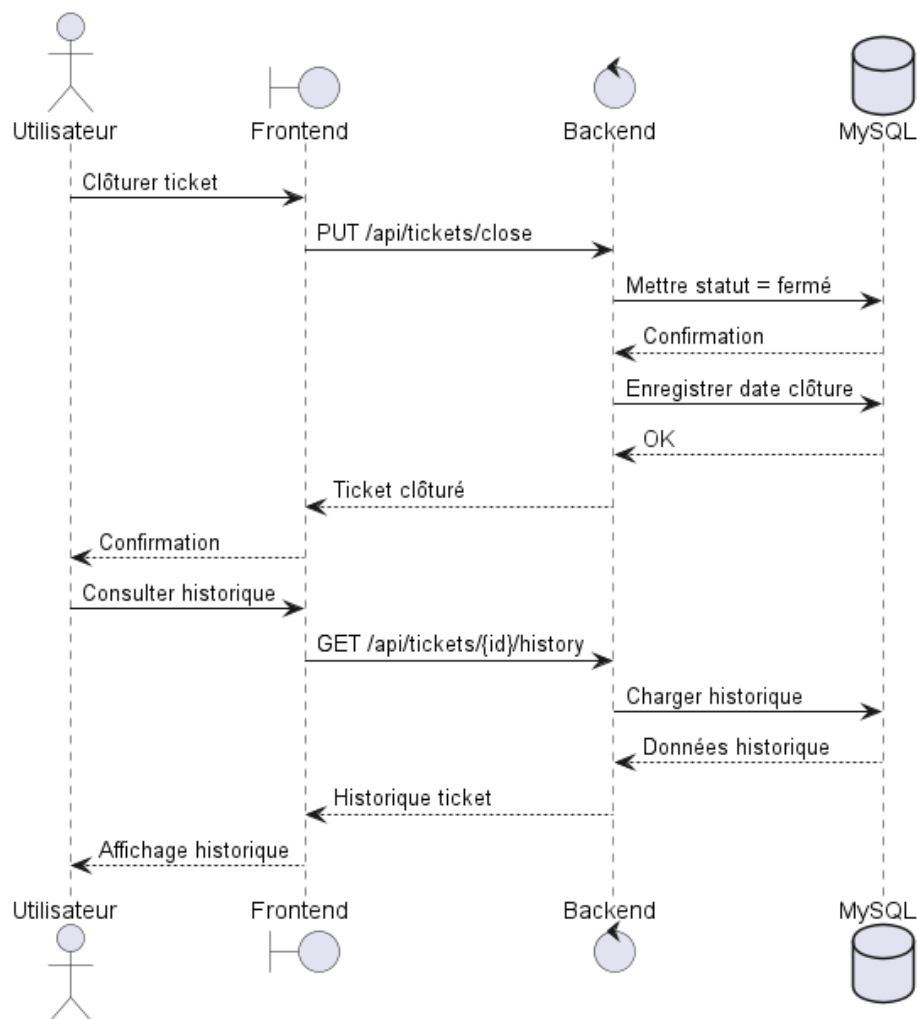
FIGURE 3.8 – Diagramme de séquence de clôture et consultation de l'historique d'un ticket
