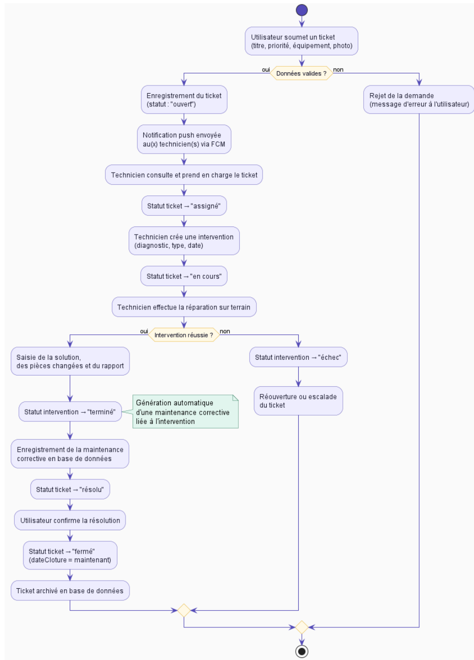
FIGURE 3.9 – Diagramme d'activité du flux des processus
